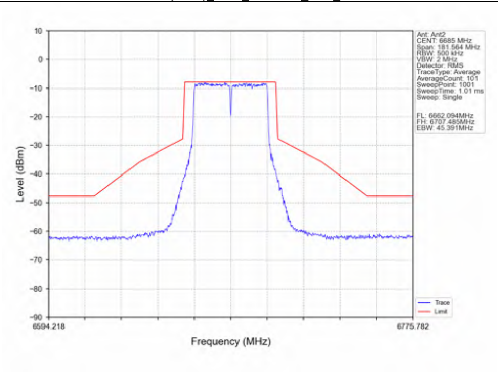
802.11n(HT40)_MCH_6685MHz_Ant2_NTNV
