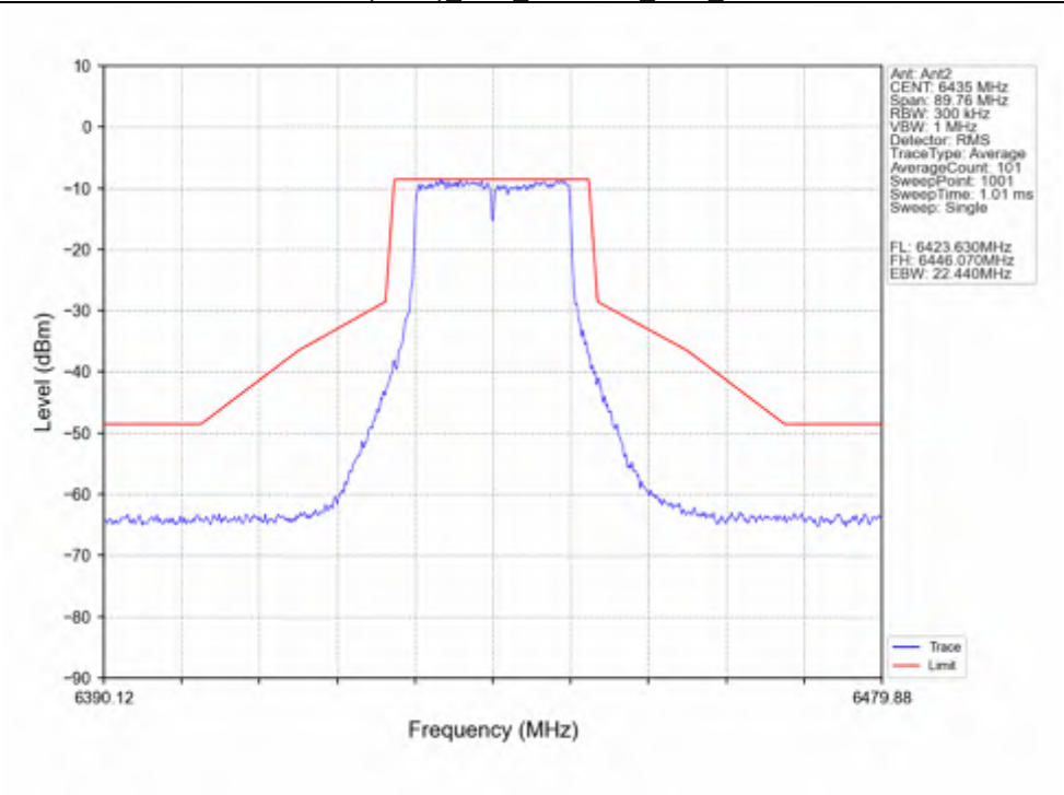
802.11n(HT20) LCH_6435MHz_Ant2_NTNV
