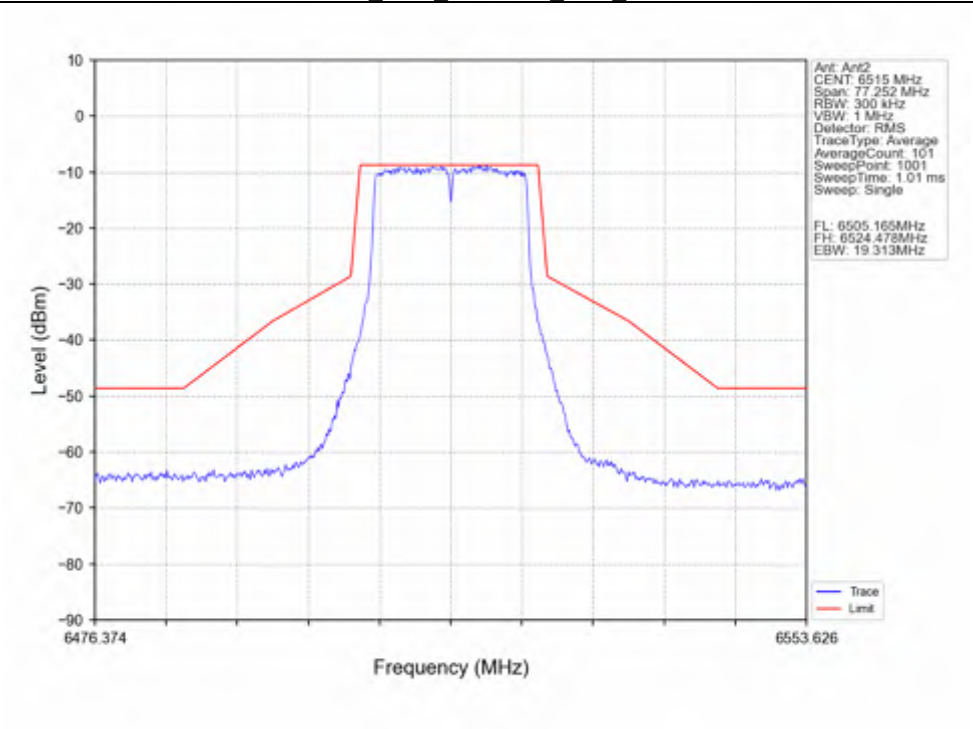
802.11a_HCH_6515MHz_Ant2_NTNV
