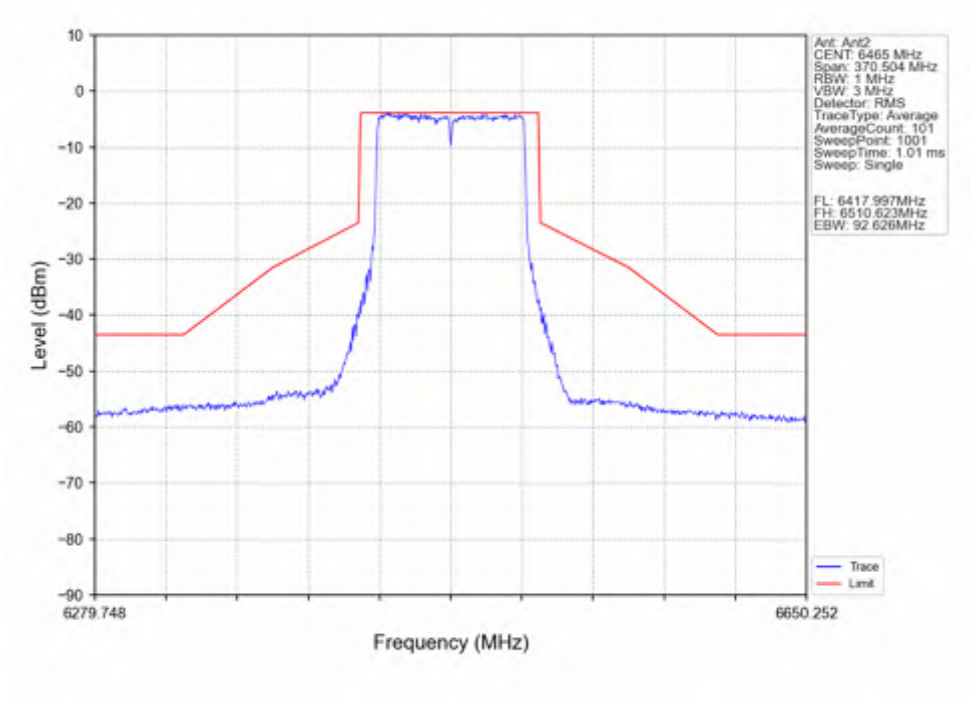
802.11ac(VHT80) LCH_6465MHz_Ant2_NTNV
