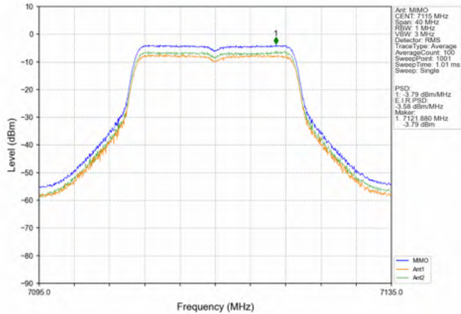
802.11n(HT20)_HCH_7115MHz_MIMO_NTNV
