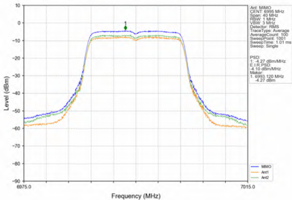
802.11a_MCH_6995MHz_MIMO_NTNV
