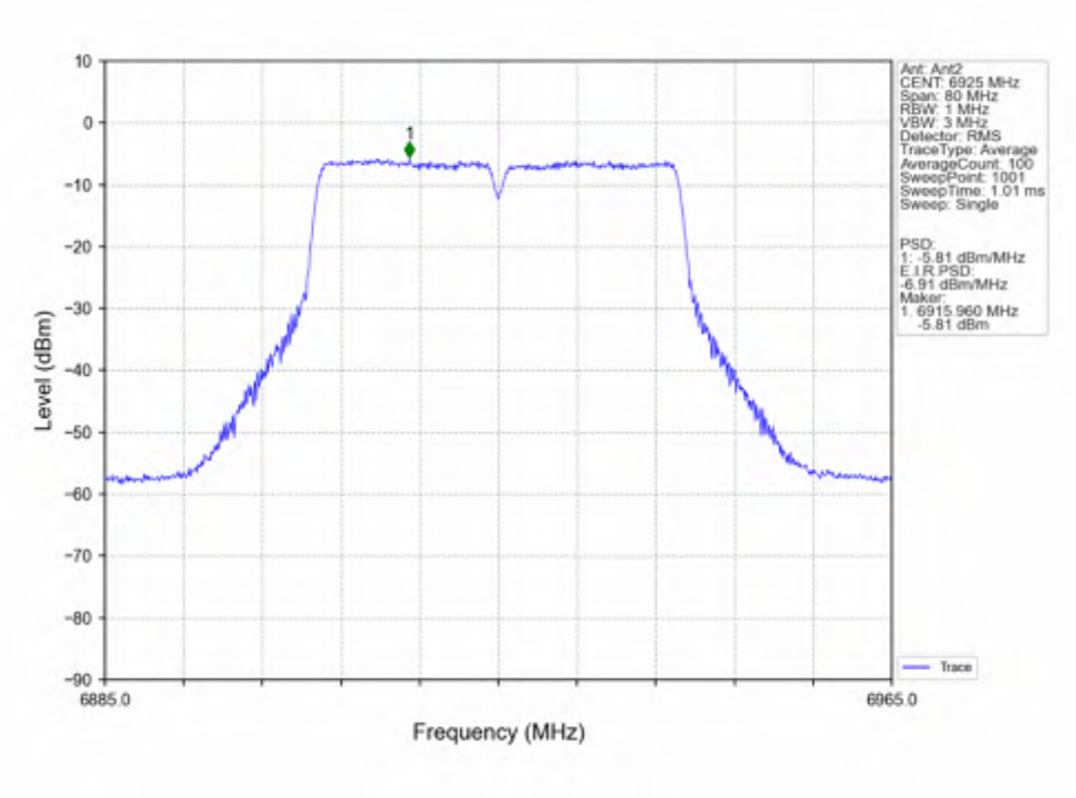
802.11ac(VHT40) LCH_6925MHz_Ant2_NTNV
