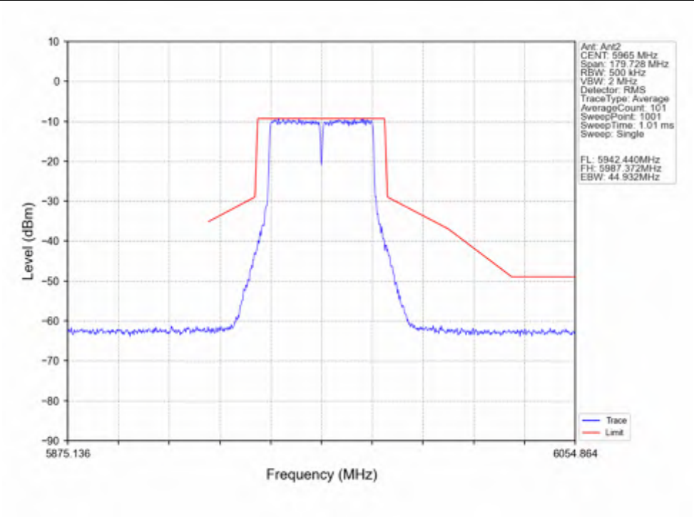
802.11ac(VHT40) LCH_5965MHz_Ant2_NTNV
