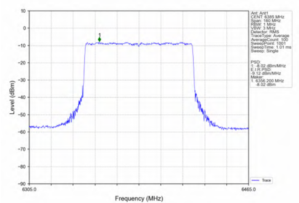
802.11ax(HEW80)_HCH_6385MHz_SU / Ant1_NTNV
