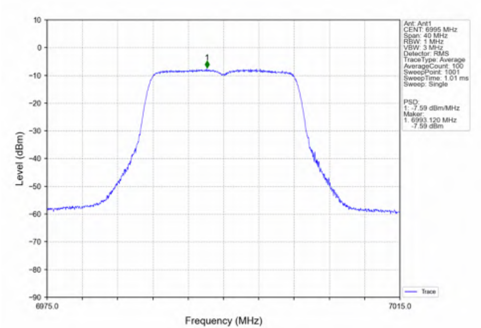
802.11a_MCH_6995MHz_Ant1_NTNV
