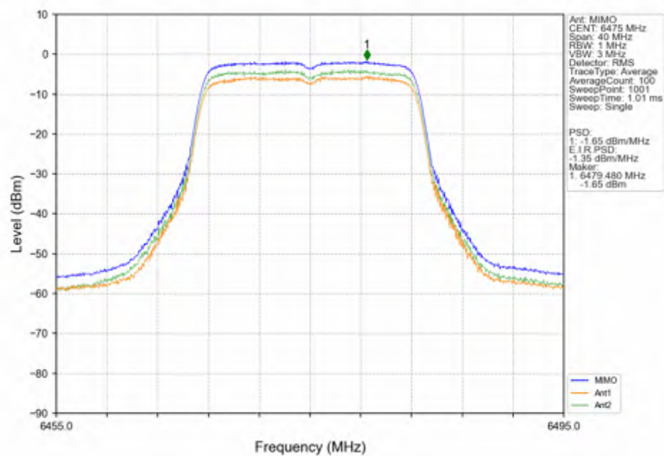
802.11a_MCH_6475MHz_MIMO_NTNV
