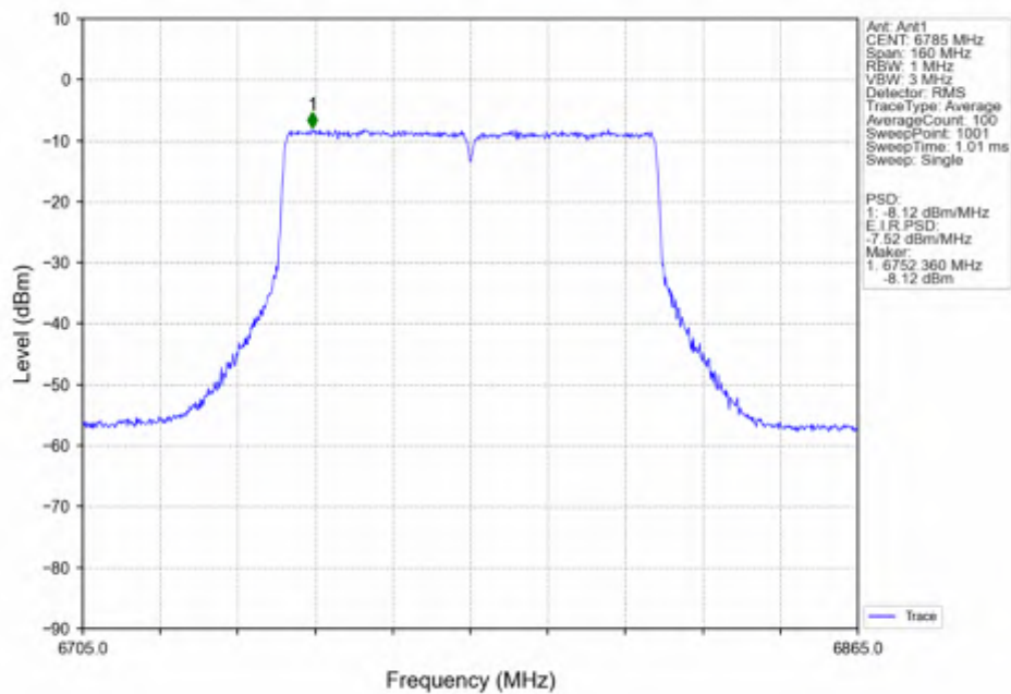
802.11ac(VHT80)_HCH_6785MHz_Ant1_NTNV
