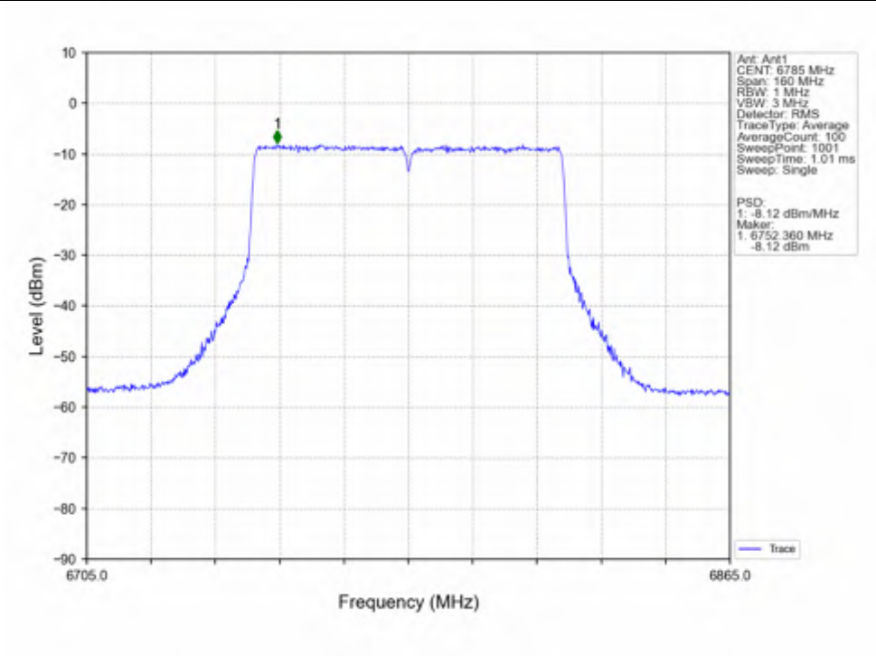
802.11ac(VHT80)_HCH_6785MHz_Ant1_NTNV
