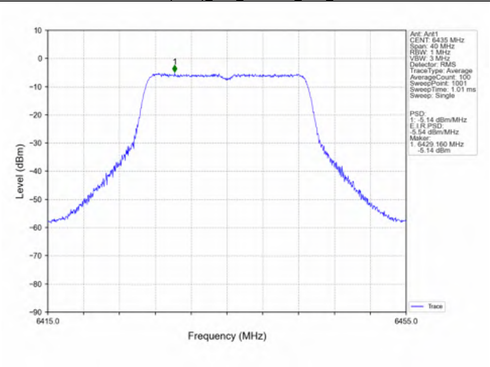
802.11n(HT20)_LCH_6435MHz_Ant1_NTNV
