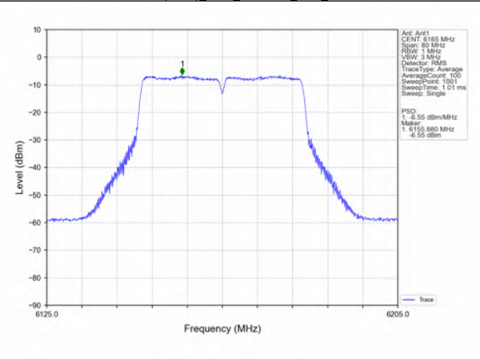
802.11n(HT40)_MCH_6165MHz_Ant1_NTNV
