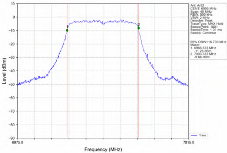
802.11a_MCH_6995MHz_Ant2_NTNV
