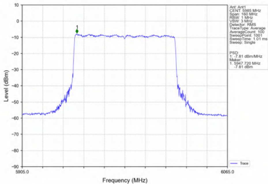
802.11ax(HEW80)_LCH_5985MHz_SU / Ant1_NTNV
