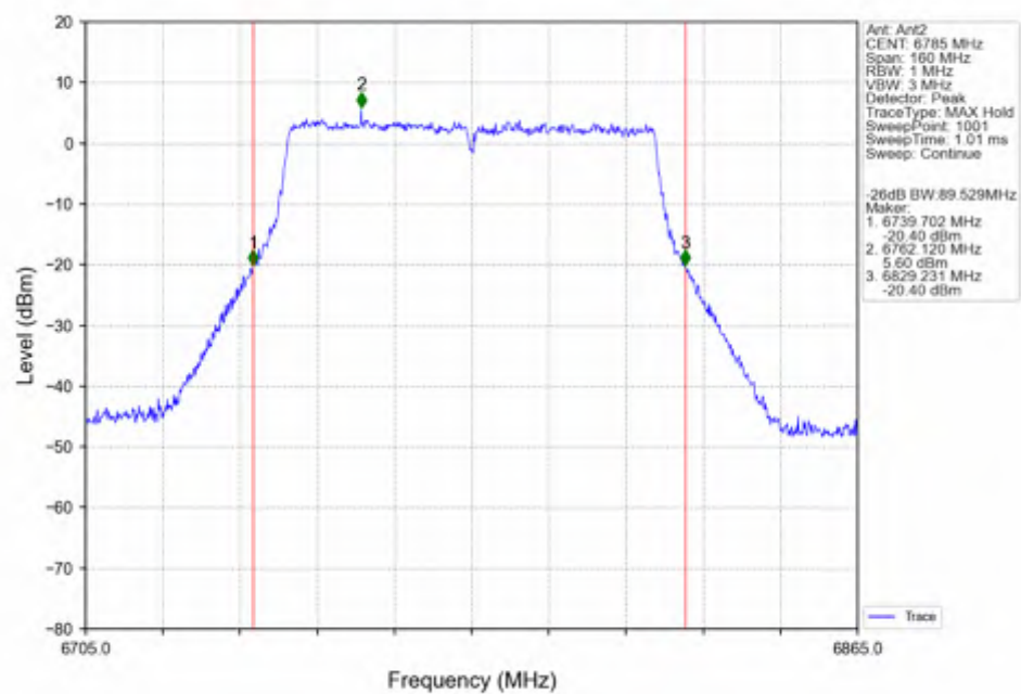
802.11ac(VHT80)_HCH_6785MHz_Ant2_NTNV
