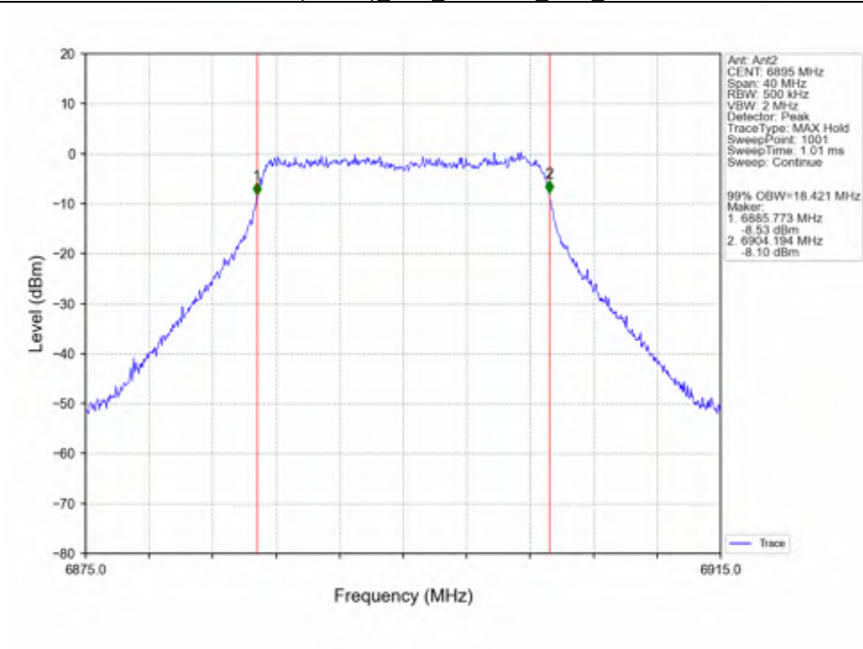
802.11ac(VHT20) LCH_6895MHz_Ant2_NTNV
