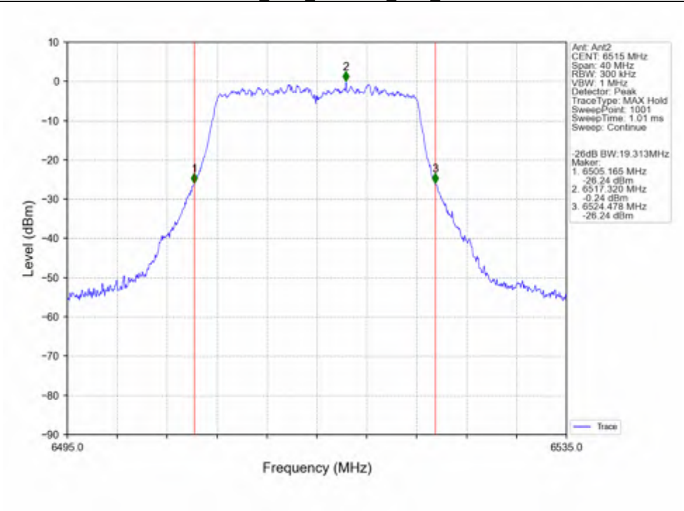
802.11a_HCH_6515MHz_Ant2_NTNV
