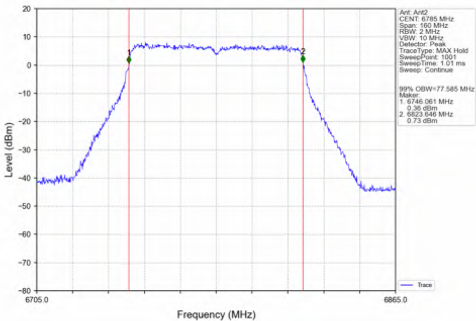
802.11ac(VHT80)_HCH_6785MHz_Ant2_NTNV
