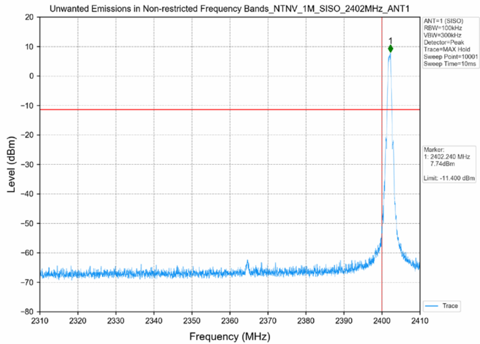
1M_2402MHz_SISO_ANT1
