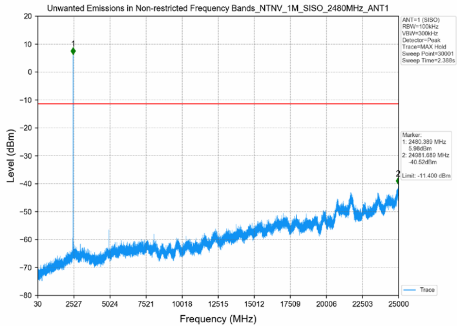
1M_2480MHz_SISO_ANT1
