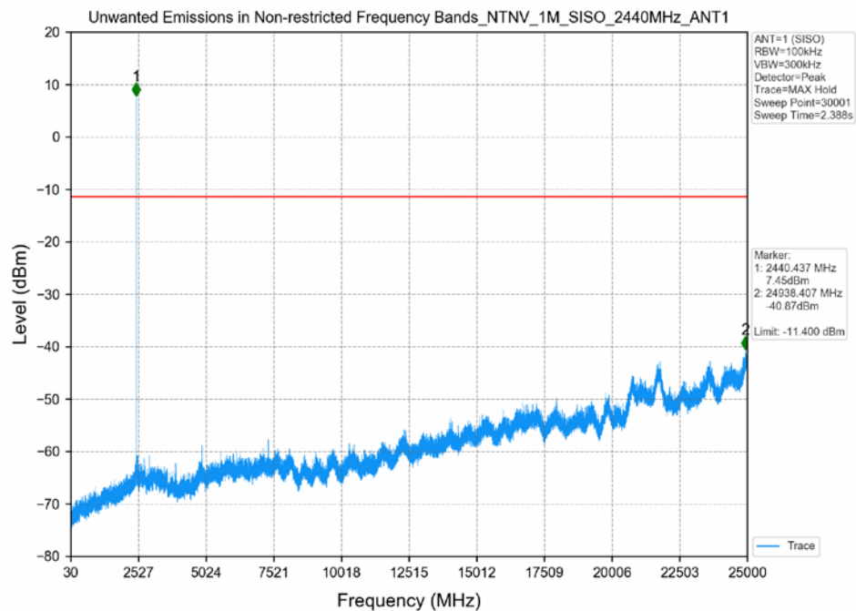
1M_2440MHz_SISO_ANT1
