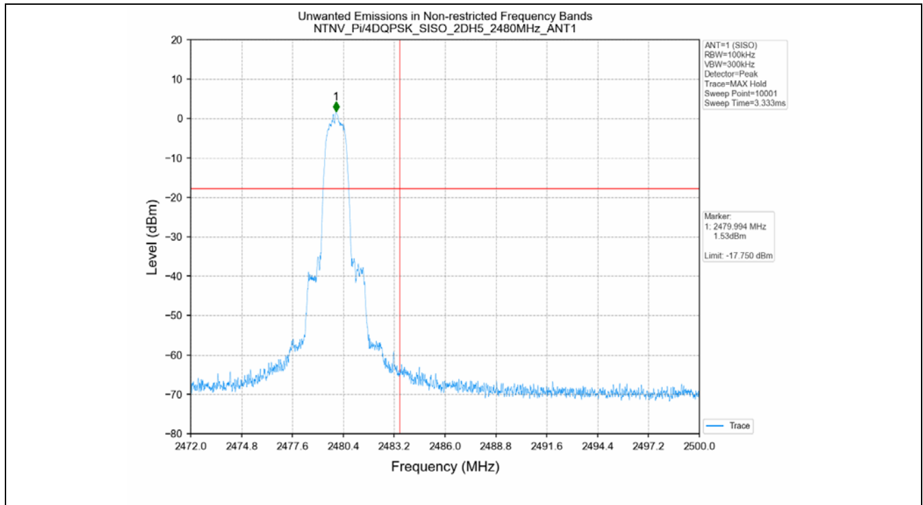
Pi/4DQPSK_2480MHz_2DH5_SISO_ANT1
