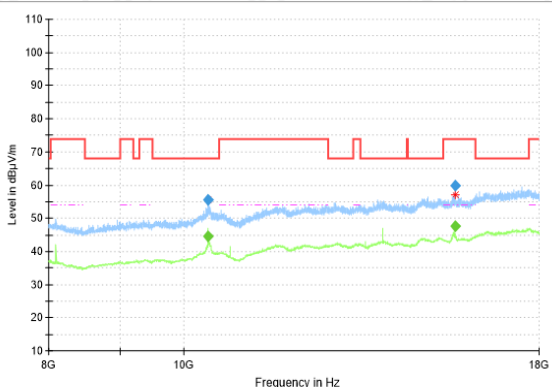
RSE-11AC(80M)-CH42-8GHz-18GHz
