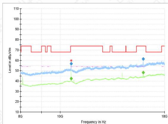
RSE-11N-CH64-8GHz-18GHz
