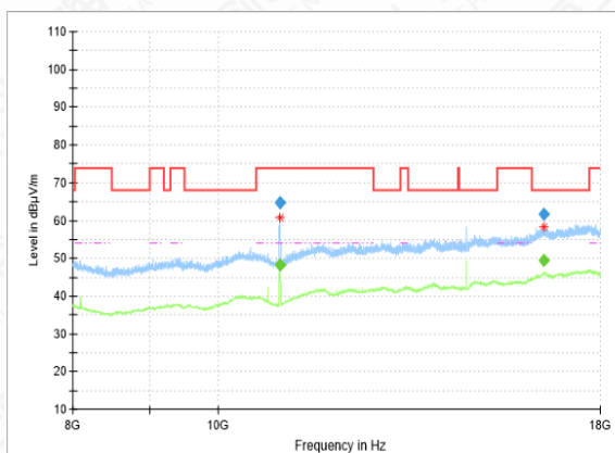
RSE-11N-CH100-8GHz-18GHz
