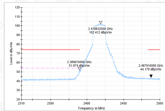
BANDEDGE-11G-CH2-AV
