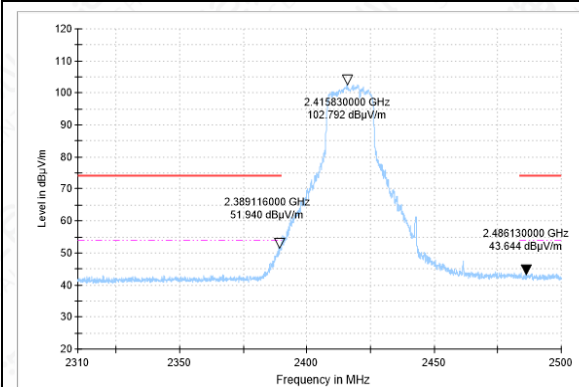
BANDEGE-11N(20M)-CH2-AV
