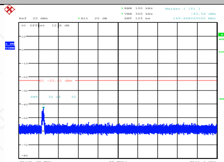
11G-Ant1-2462-30~1000-PASS
