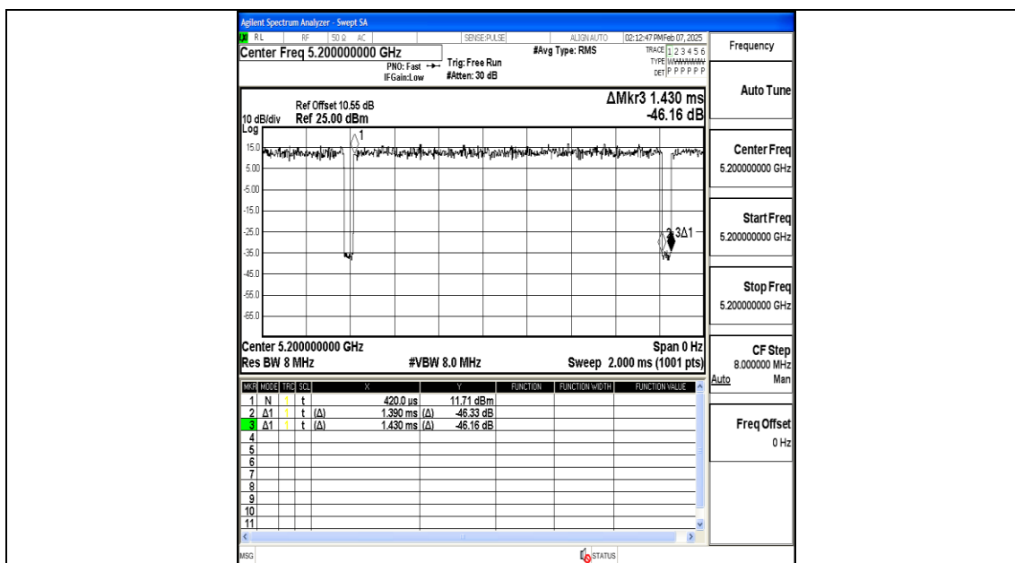
NTNV-11A-Ant1-5200
