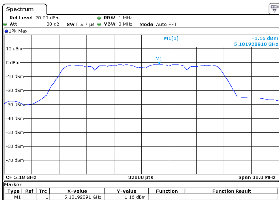
Ant 802.11 a
