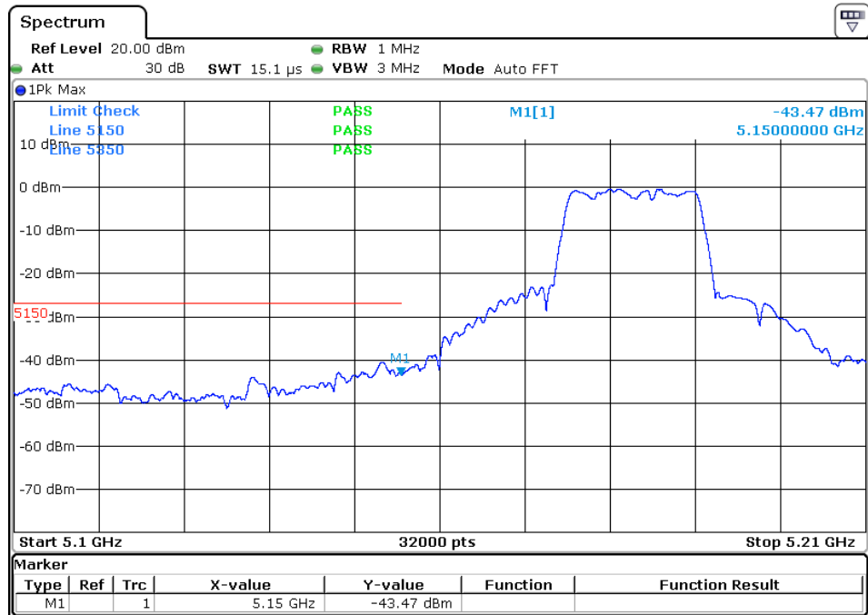
Ant 802.11 a
