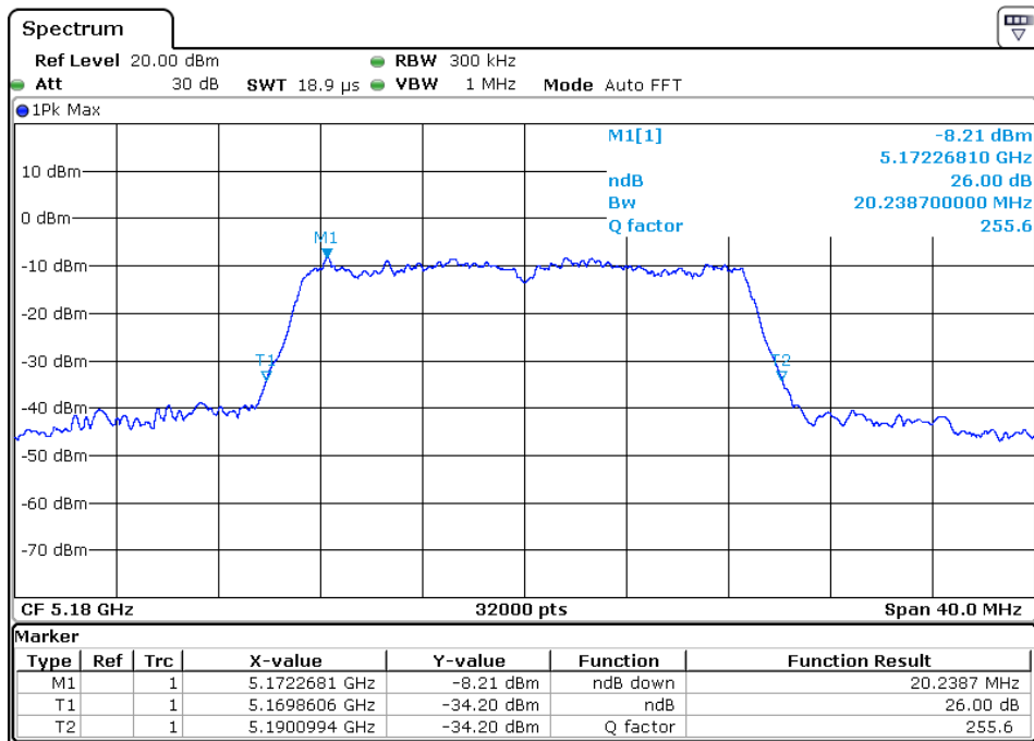
Ant 802.11 a
