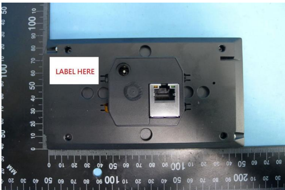
(8) EUT Photo (Opus, Opus XL)
