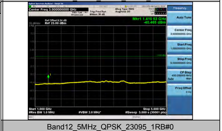
Band12 5MHz QPSK 23095 1RB#0
