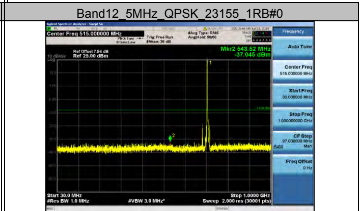
Band12 5MHz QPSK 23155 1RB#0
