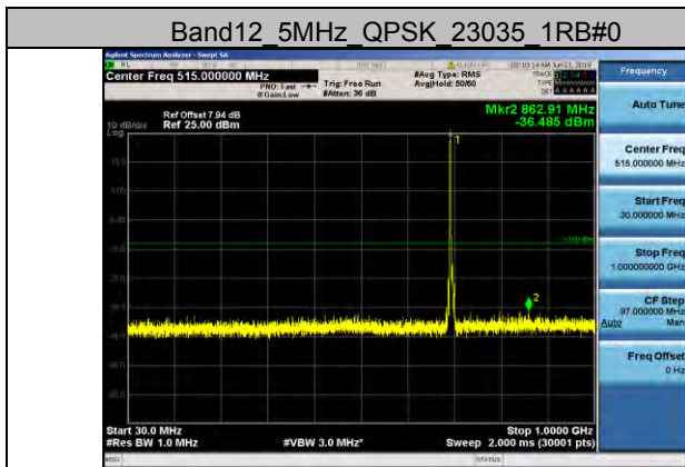
Band12 5MHz QPSK 23035 1RB#0
