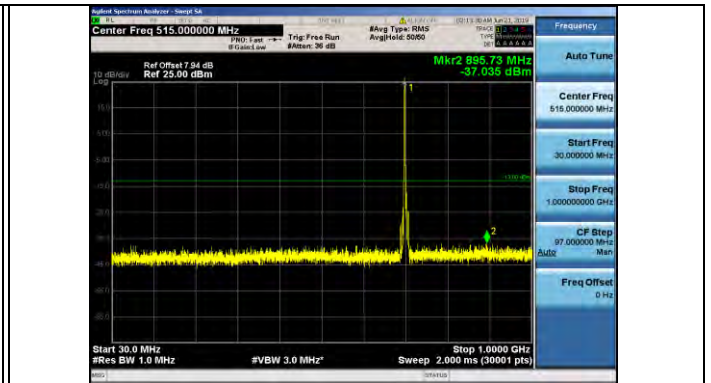
Band12 5MHz QPSK 23095 1RB#0
