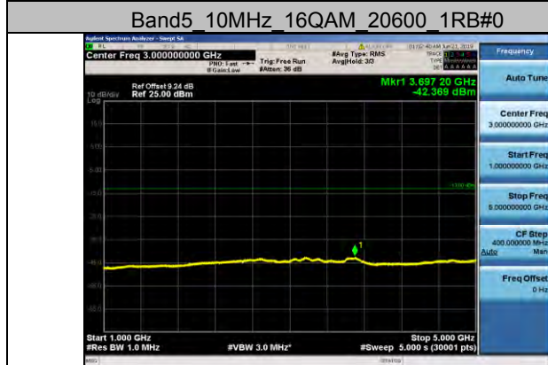
Band5 10MHz 16QAM 20600 1RB#0
