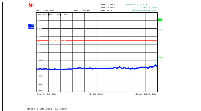
Band7_20MHz_16QAM_21350_1RB#0
