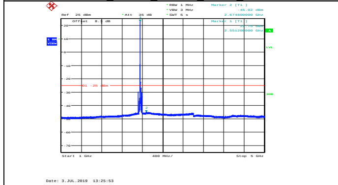
Band7_20MHz_16QAM_21350_1RB#0
