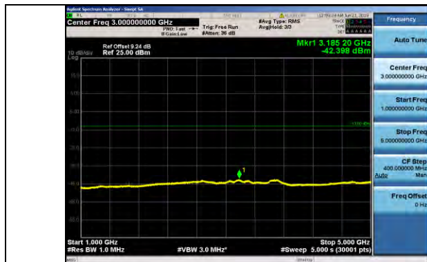
Band5 10MHz 16QAM 20525 1RB#0
