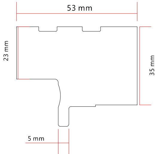
尺寸图 A-图
