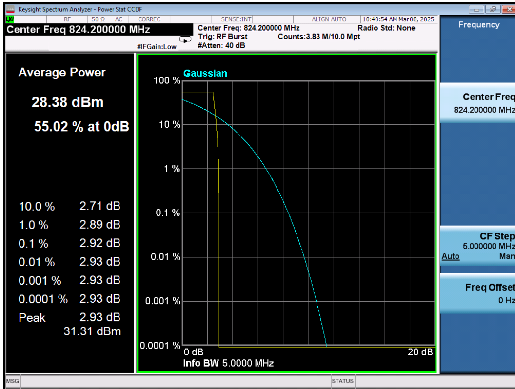
GSM850\GPRS\L
