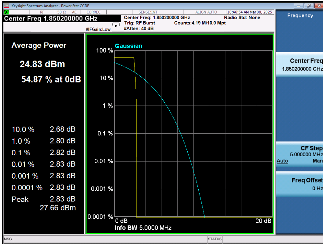
GSM1900\GSM\L
