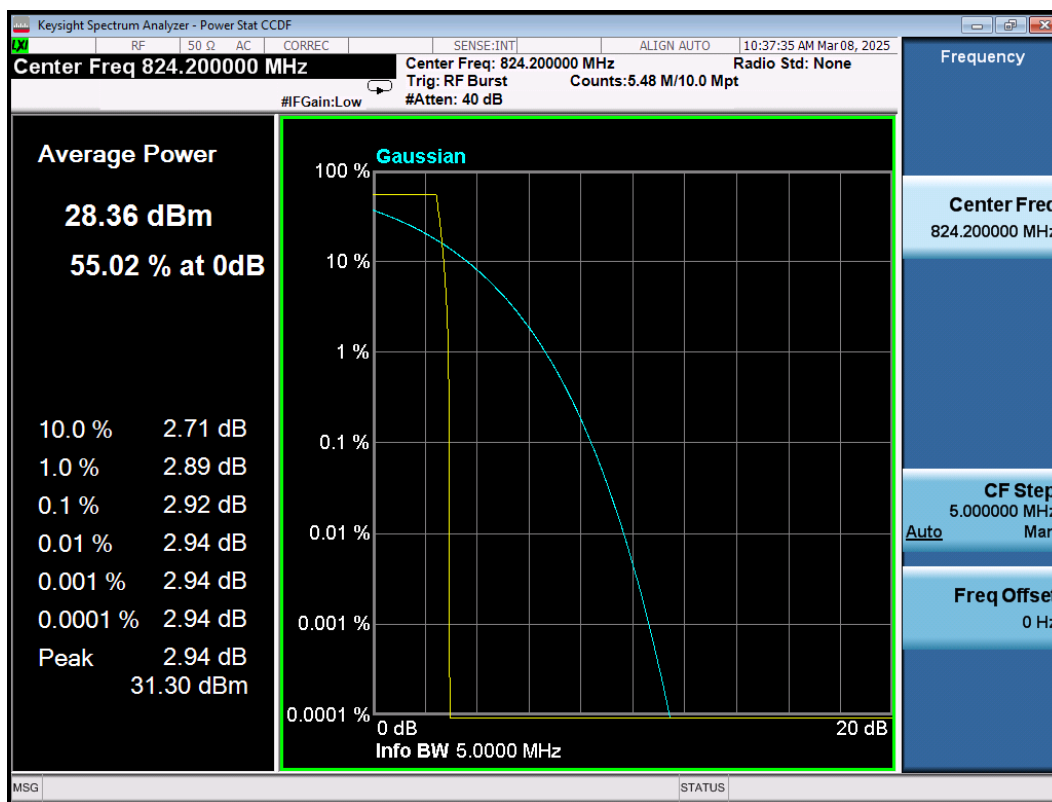
GSM850\GSM\L
