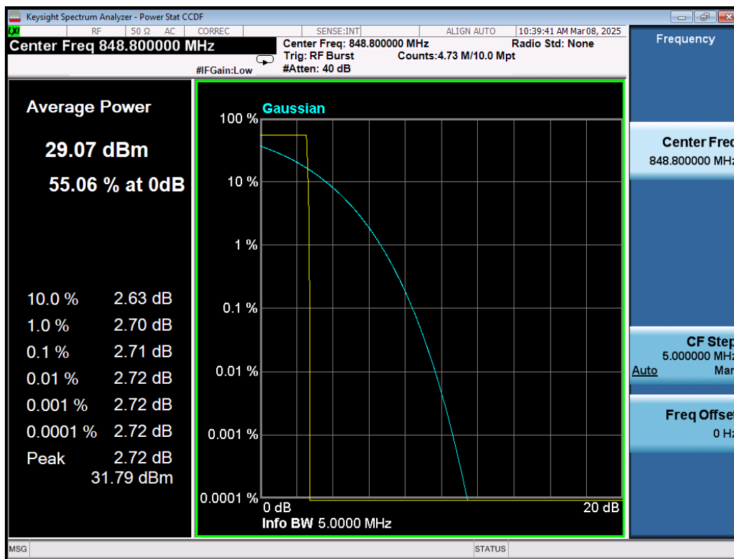
GSM850\GSM\H
