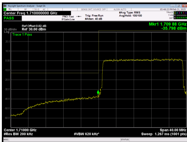
LLTE Band66 QAM64 BW=20MHz Channel=132072 RB Size=100 Position=#0
