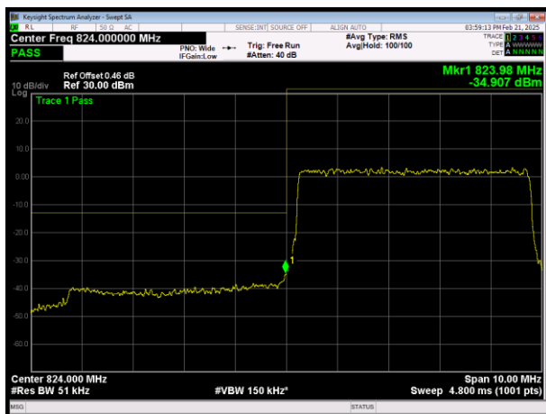
LLTE Band5 QAM64 BW=5MHz Channel=20425 RB Size=25 Position=#0
