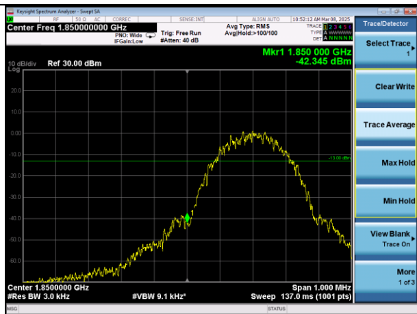
GSM1900\EGPRS\I
