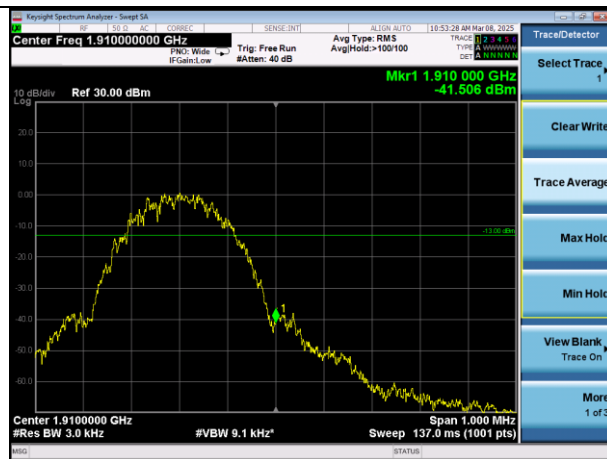
GSM1900\EGPRS\H
