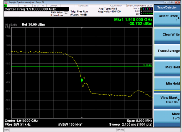
WCDMA B2/H
