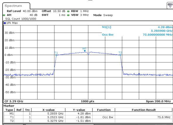
802.11ac80_5290MHz
