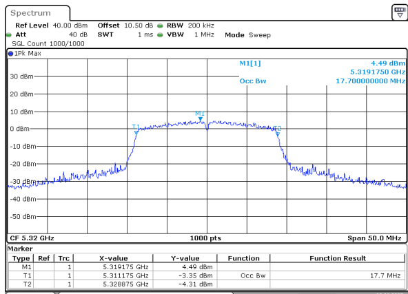
802.11n20_5320MHz
