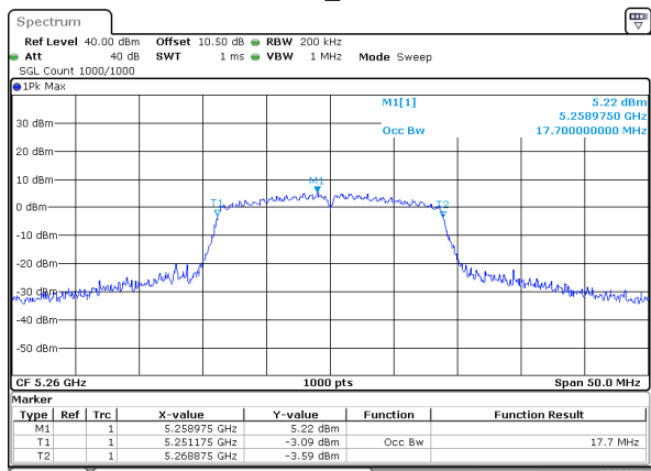
802.11n20_5260MHz
