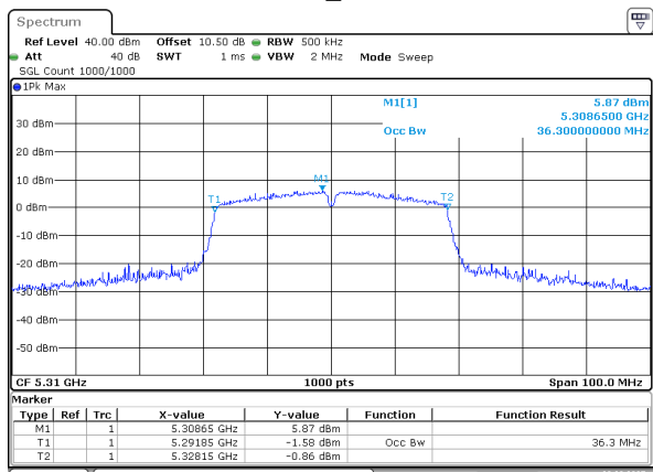
802.11n40_5310MHz
