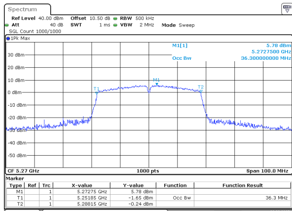
802.11n40_5270MHz
