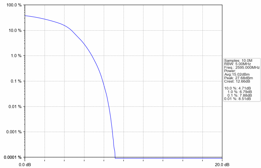
Band41_10MHz_16QAM_MCH_2595MHz_RB_50_0_NTNV
