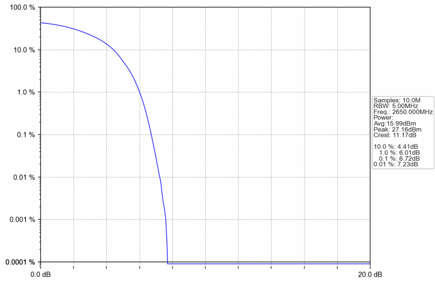
Band41_10MHz_QPSK_HCH_2650MHz_RB_50_0_NTNV
