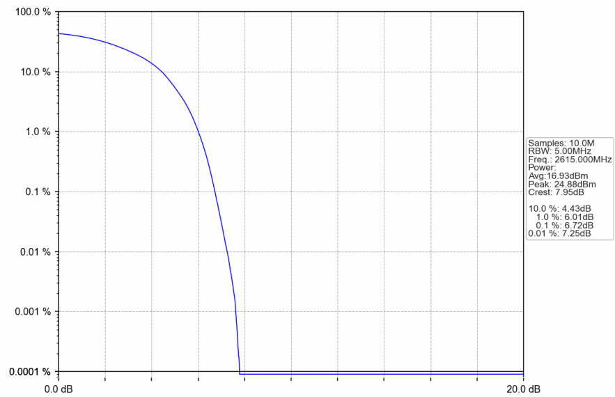
Band38_10MHz_QPSK_HCH_2615MHz_RB_50_0_NTNV
