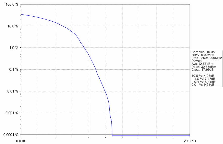
Band41_20MHz_16QAM_MCH_2595MHz_RB_100_0_NTNV
