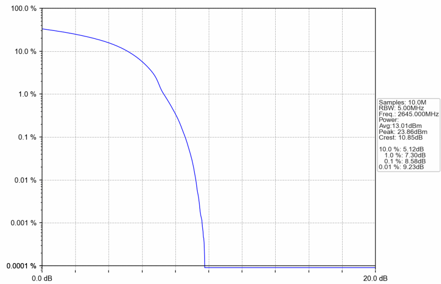
Band41_20MHz_QPSK_HCH_2645MHz_RB_100_0_NTNV
