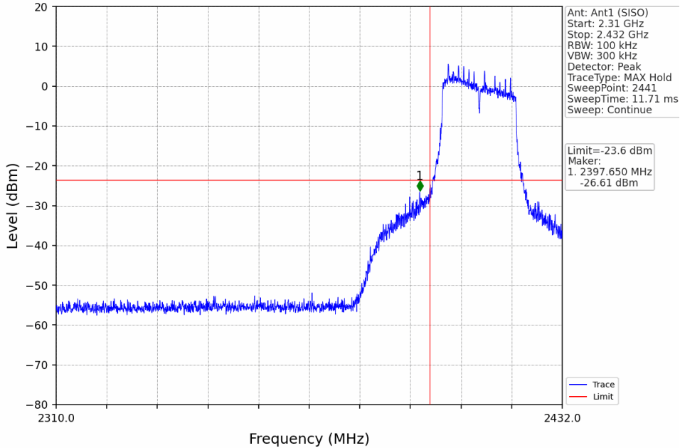
802.11n(HT20)_LCH_2412MHz_Ant1 (SISO)_NTNV
