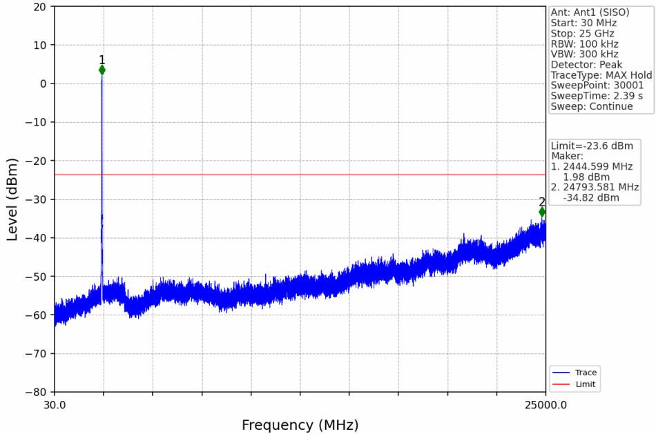
802.11n(HT20)_HCH_2462MHz_Ant1 (SISO)_NTNV
