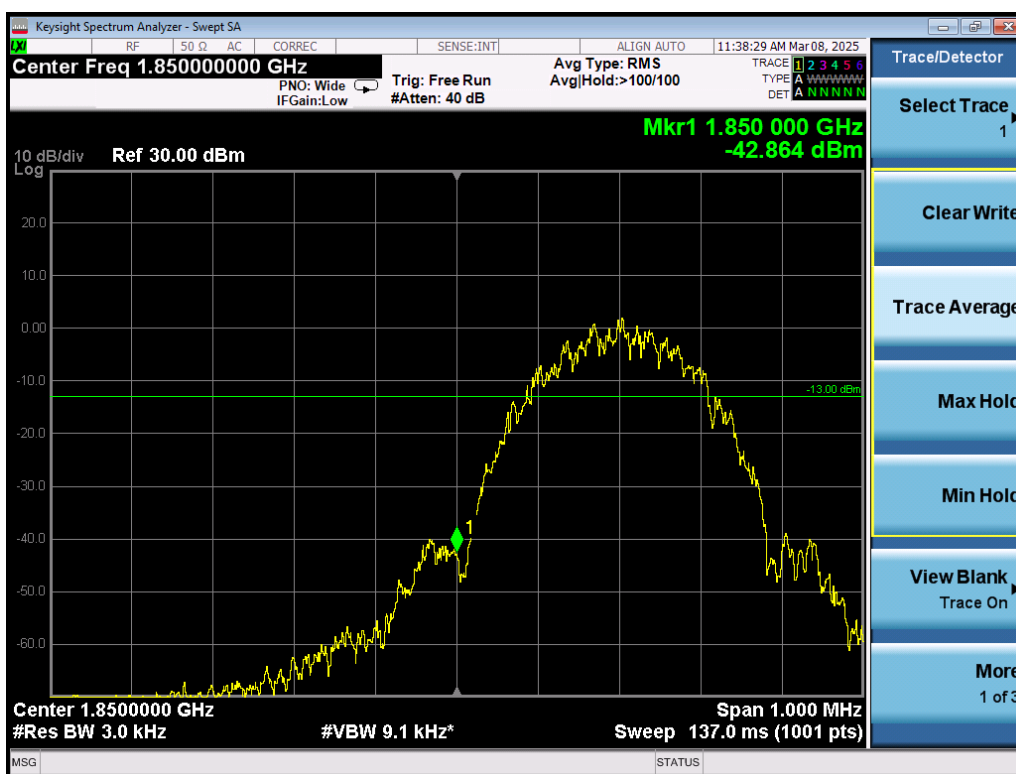
GSM1900\EGPRS\L
