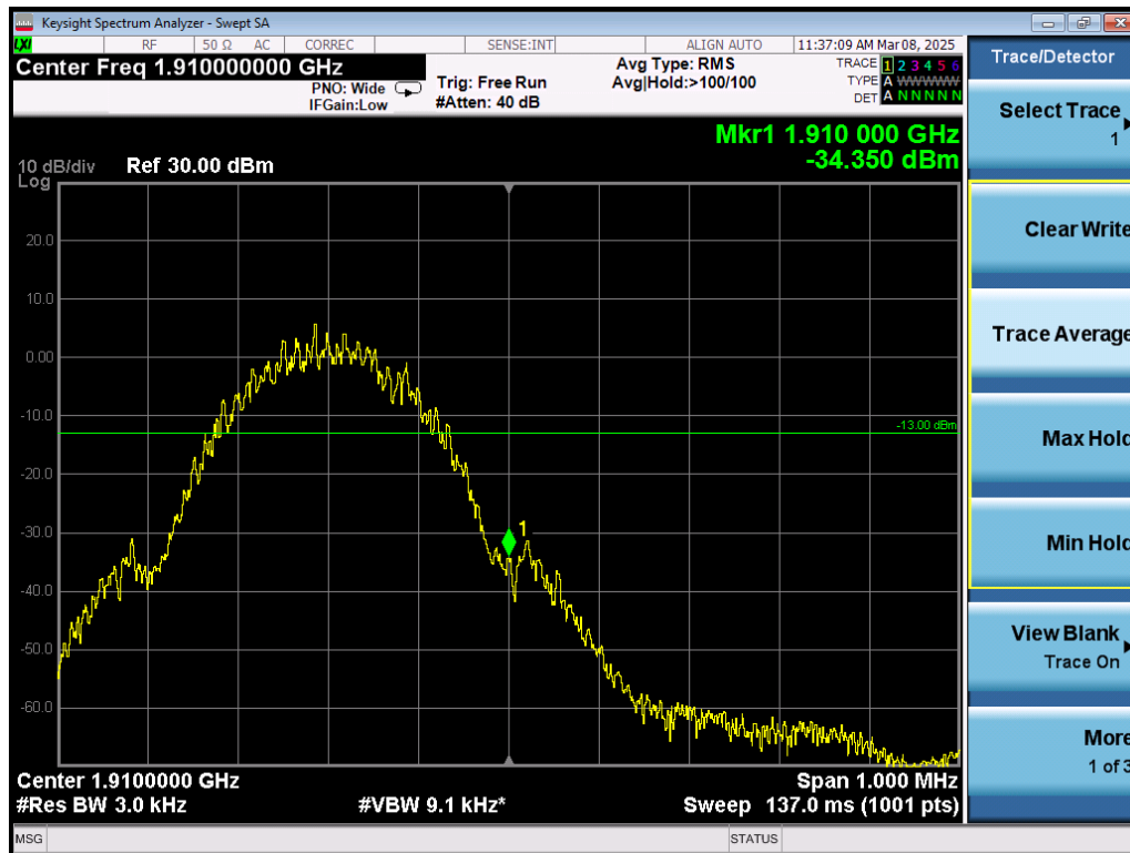
GSM1900\GPRS\H
