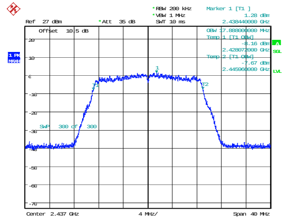
802.11n20_2437MHz_Chain 0
