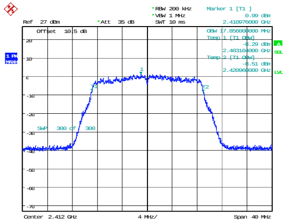
802.11n20_2412MHz_Chain 0
