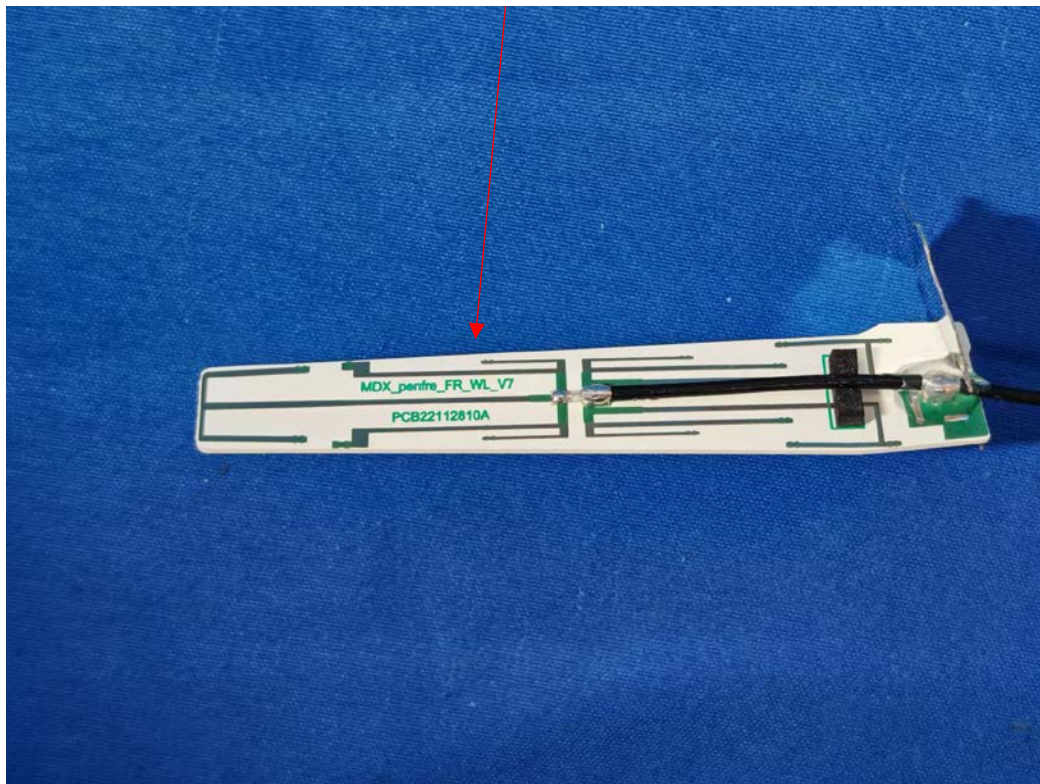
SRD ANT 1(Chain 0)
