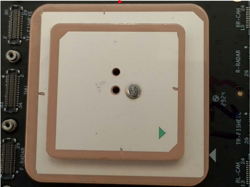
GPS Antenna
