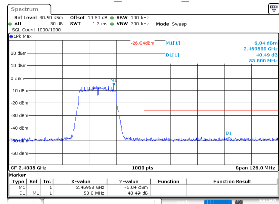
802.11n20_2462MHz_Chain 1
