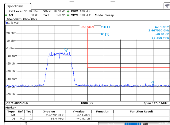
802.11n20_2462MHz_Chain 0
