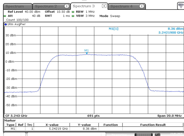
10M_5243MHz
