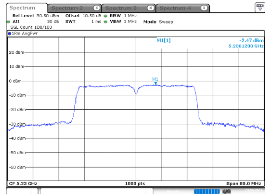
ac40_5230MHz_Chain 1
