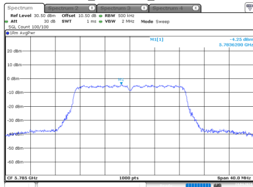
ac20_5785MHz_Chain 0
