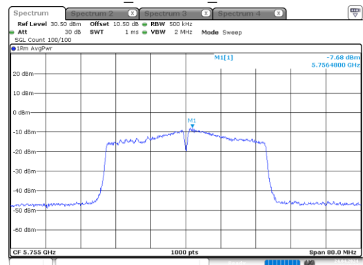
n40_5755MHz_Chain 1
