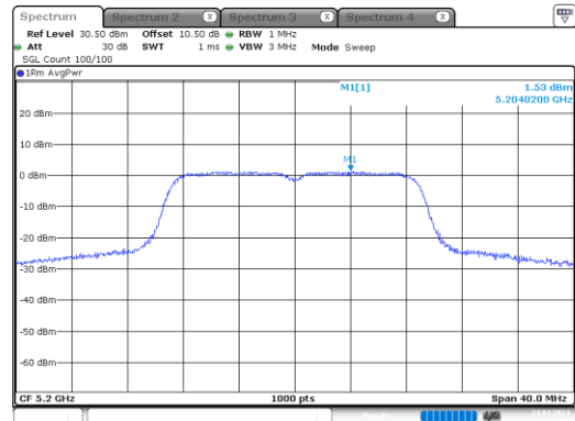
ac20_5200MHz_Chain 1
