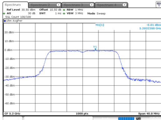
ac20_5200MHz_Chain 0
