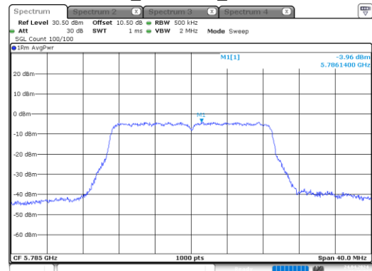
ac20_5785MHz_Chain 1
