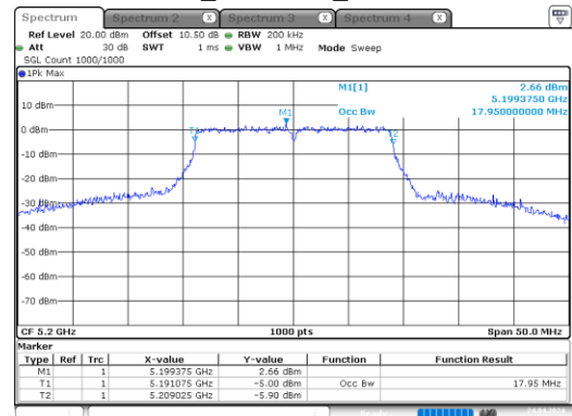
ac20_5200MHz_Chain 0
