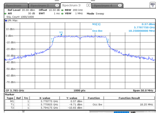
ac20_5785MHz_Chain 0
