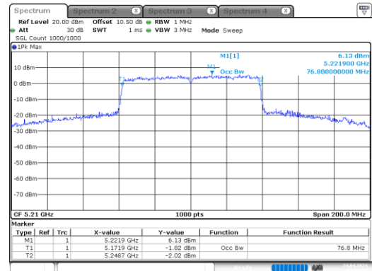
ac80_5210MHz_Chain 0
