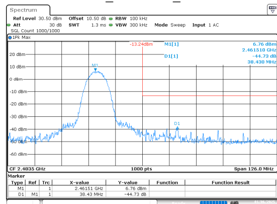
802.11b_2462MHz_Chain 1
