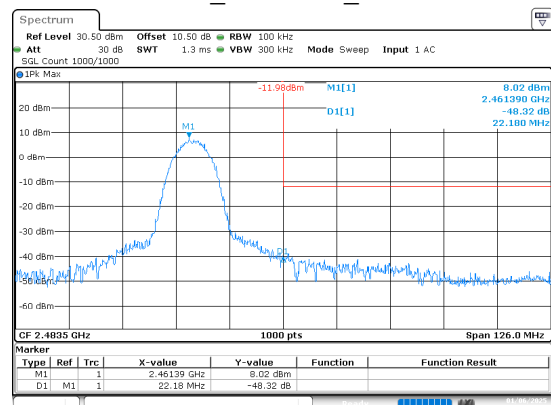
802.11b_2462MHz_Chain 0
