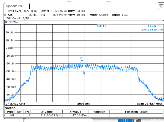
802.11n20_2412MHz_Chain 1
