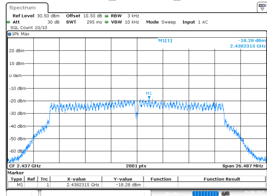
802.11n20_2437MHz_Chain 0
