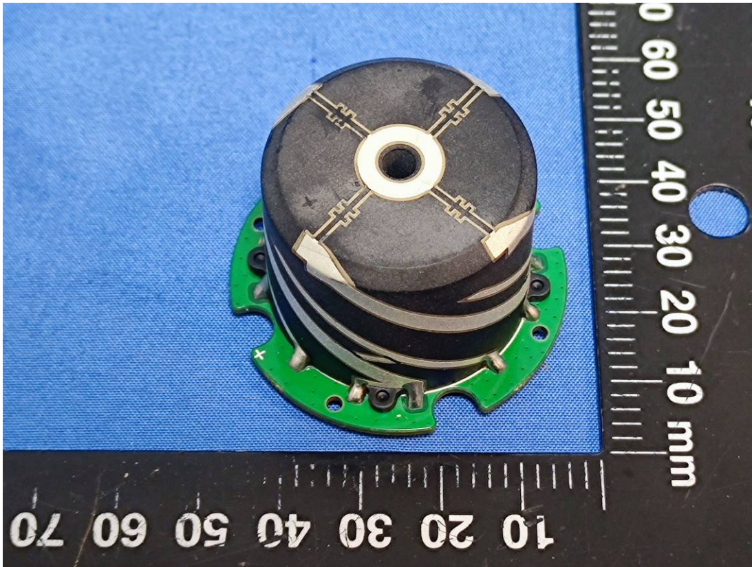
GPS Antenna
