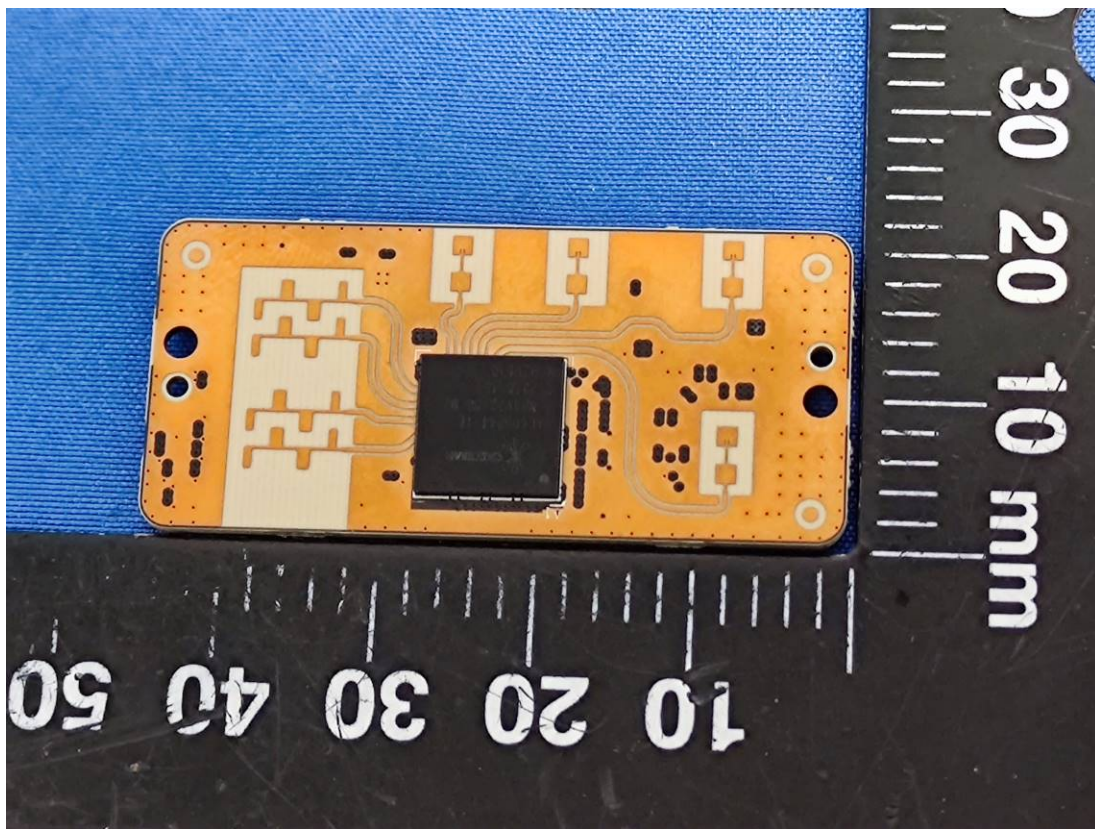
Chip&Antenna
