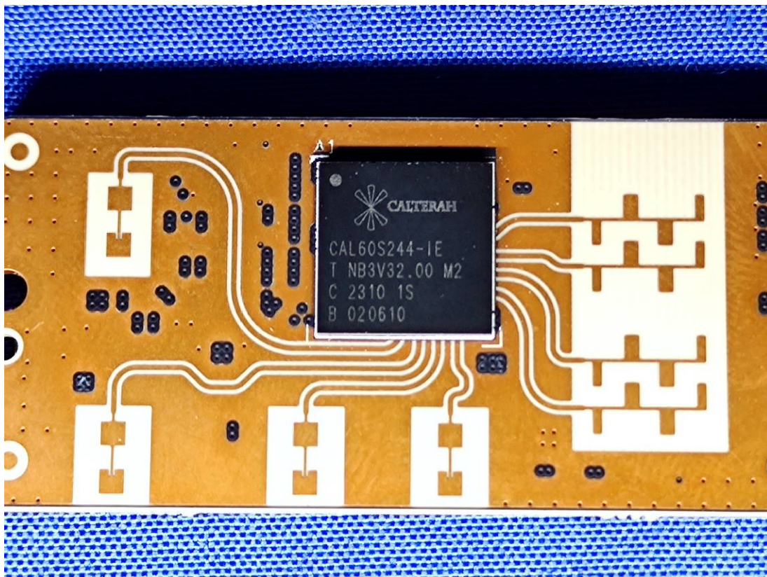
Chip&Antenna
