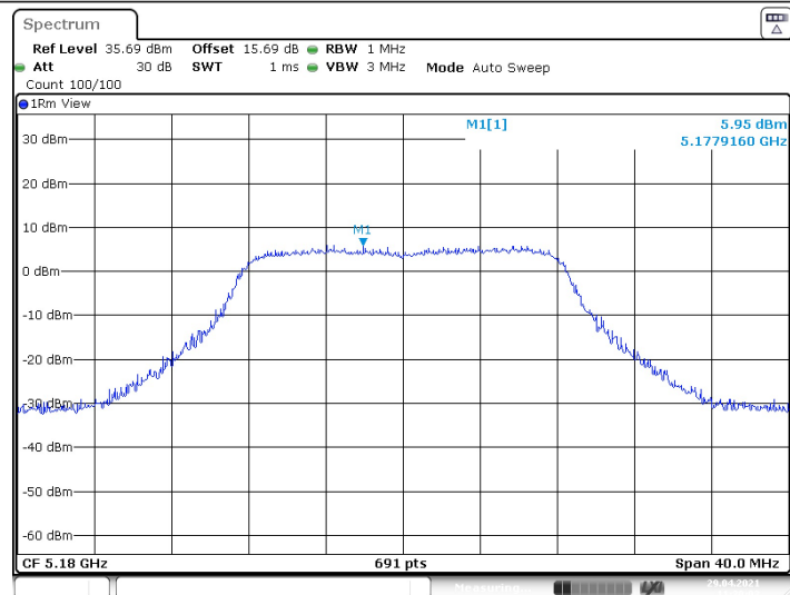
11AMIMO_Ant2_5180
