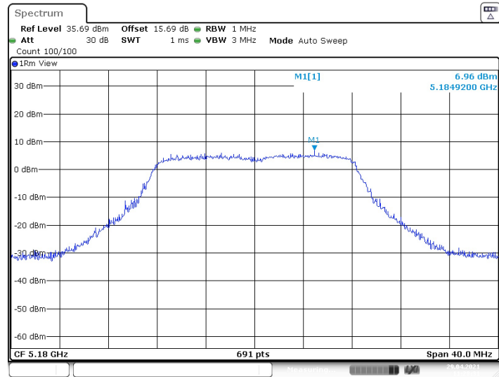
11AMIMO_Ant1_5180
