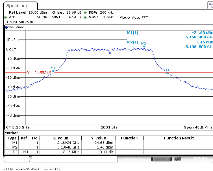
11AMIMO_Ant2_5180
