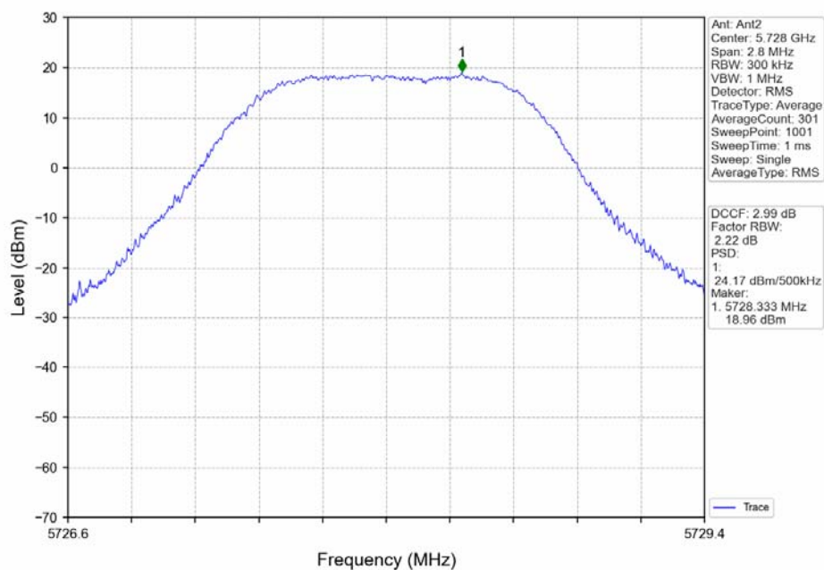
QPSK_LCH_5728MHz_Ant2_NTNV
