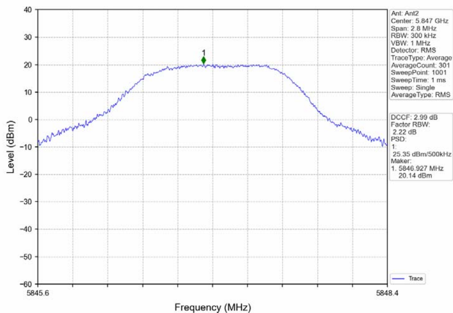
16QAM_HCH_5847MHz_MIMO_NTNV
