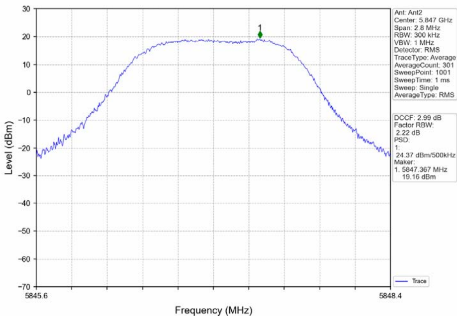
QPSK_HCH_5847MHz_Ant2_NTNV
