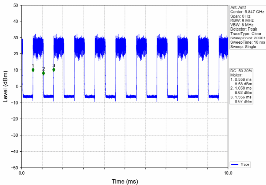
QPSK_HCH_5847MHz_Ant1_NTNV
