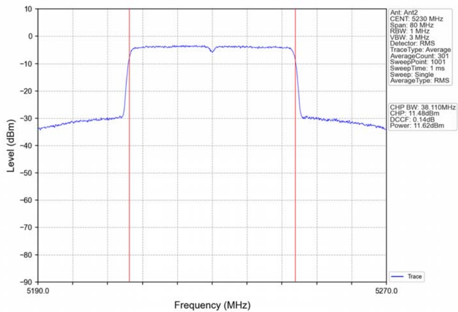
802.11ax(HEW40)_HCH_5230MHz_RU484_Left_Ant2_NTNV
