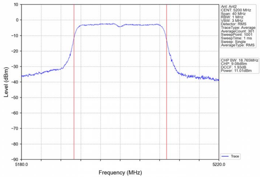
802.11n(HT20)_MCH_5200MHz_Ant2_NTNV
