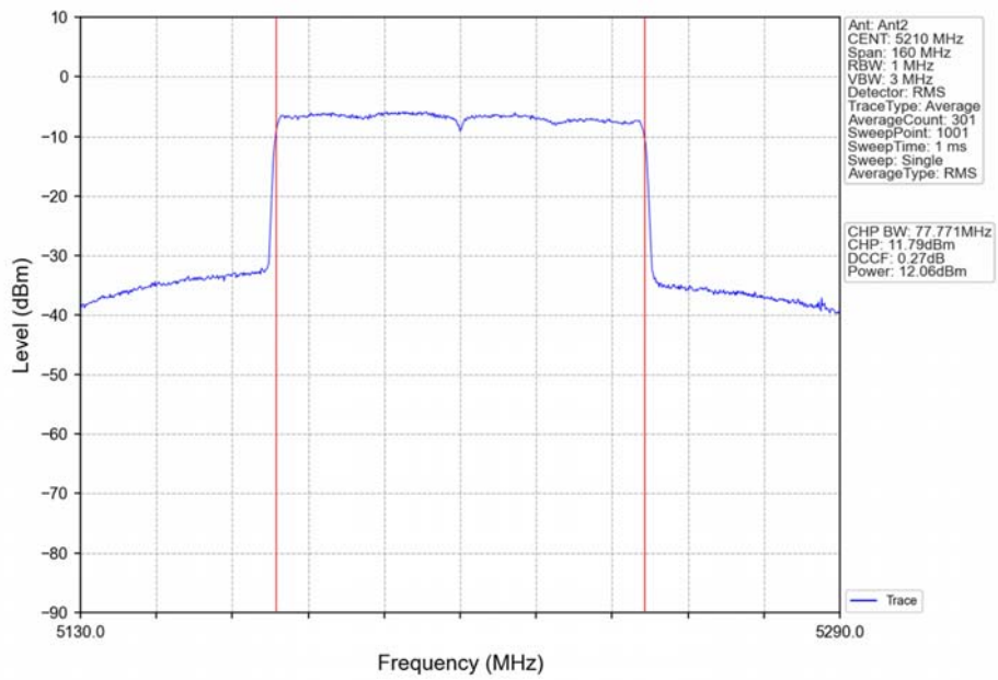
802.11ax(HEW80)_MCH_5210MHz_RU996_Left_Ant2_NTNV
