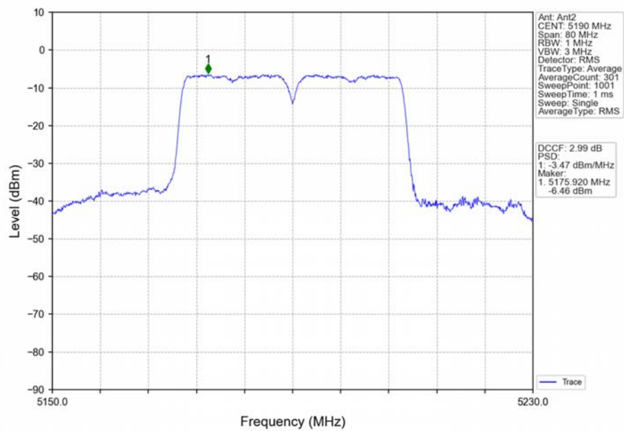
802.11n(HT40)_LCH_5190MHz_Ant2_NTNV
