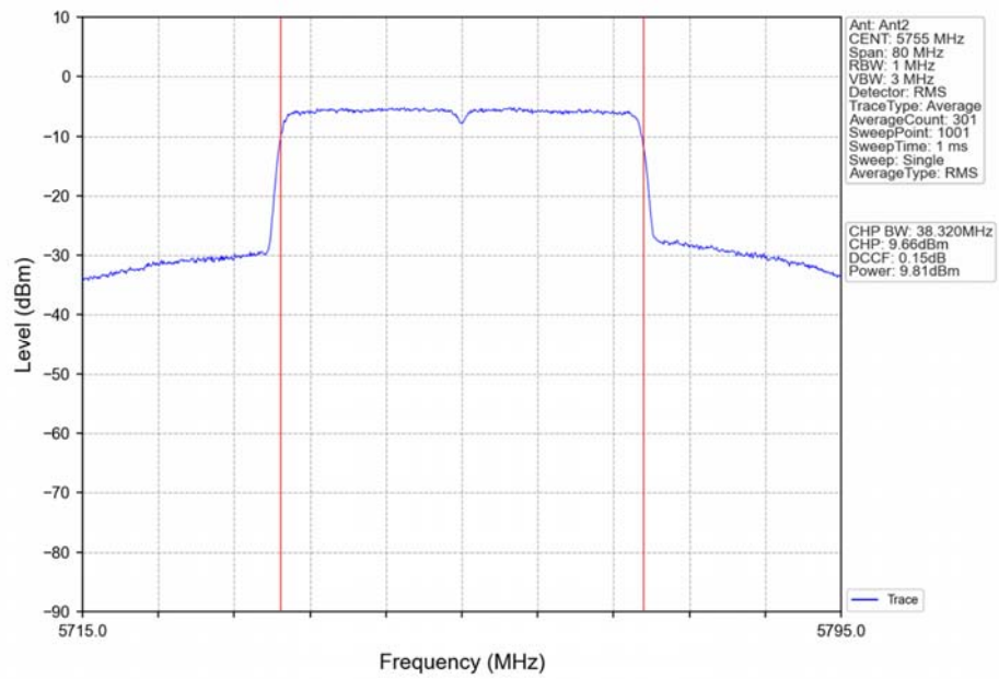
802.11ax(HEW40)_LCH_5755MHz_RU484_Left_Ant2_NTNV
