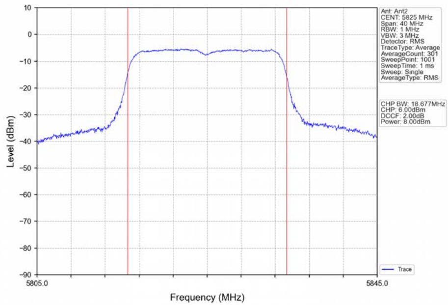
802.11n(HT20)_HCH_5825MHz_Ant2_NTNV
