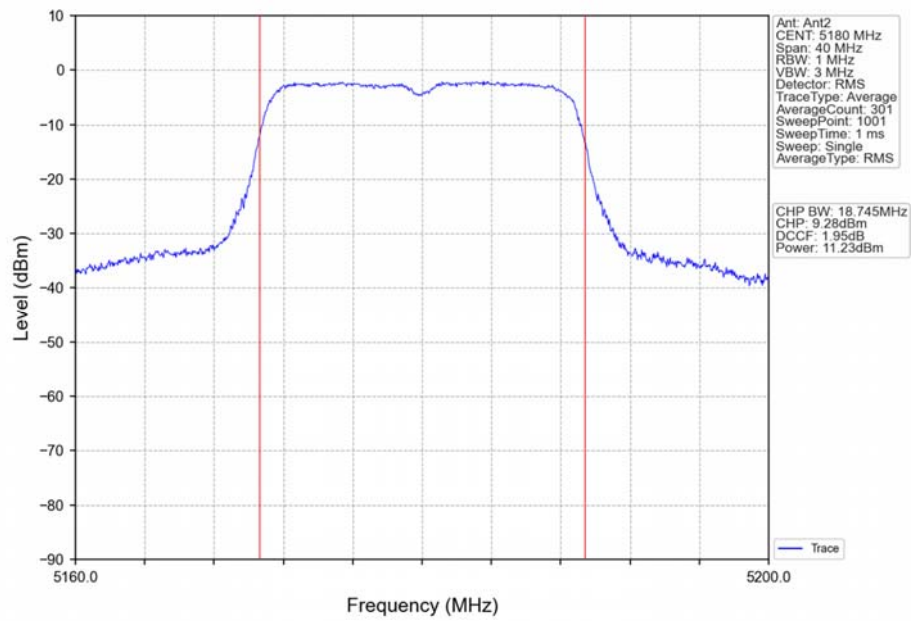
802.11n(HT20)_LCH_5180MHz_Ant2_NTNV
