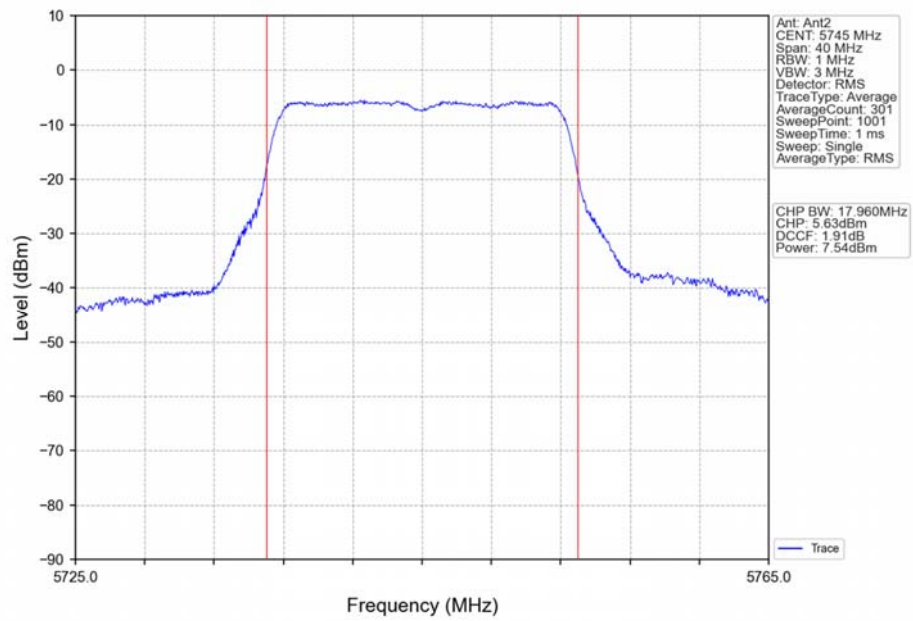
802.11a_LCH_5745MHz_Ant2_NTNV
