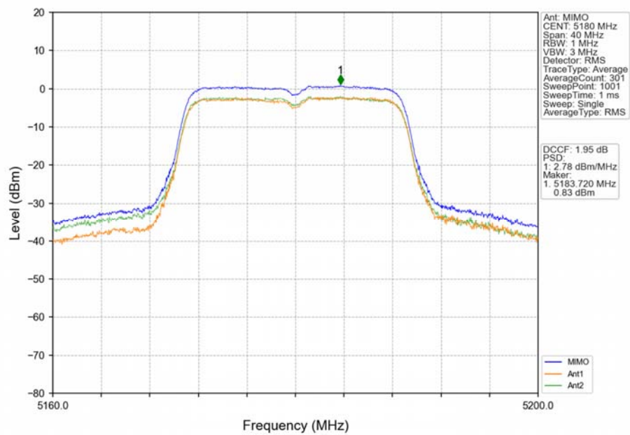
802.11n(HT20)_LCH_5180MHz_MIMO_NTNV
