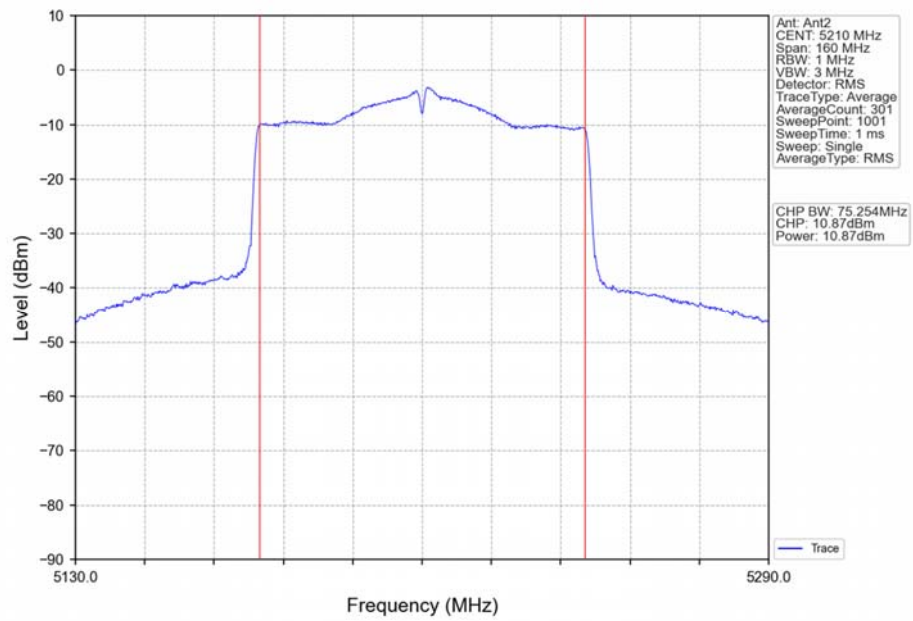
802.11ac(VHT80)_MCH_5210MHz_Ant2_NTNV
