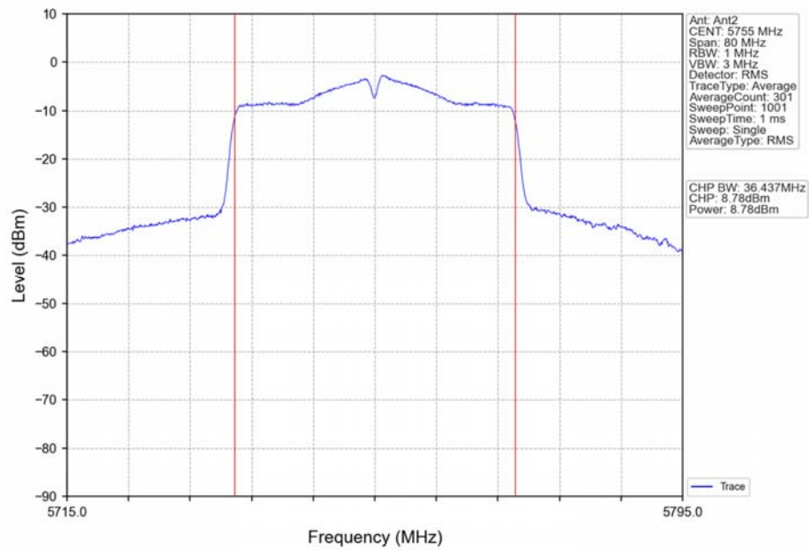
802.11ac(VHT40)_LCH_5755MHz_Ant2_NTNV
