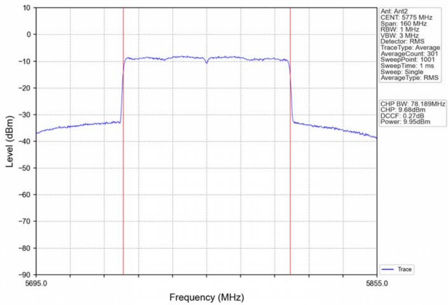
802.11ax(HEW80)_MCH_5775MHz_RU996_Left_Ant2_NTNV
