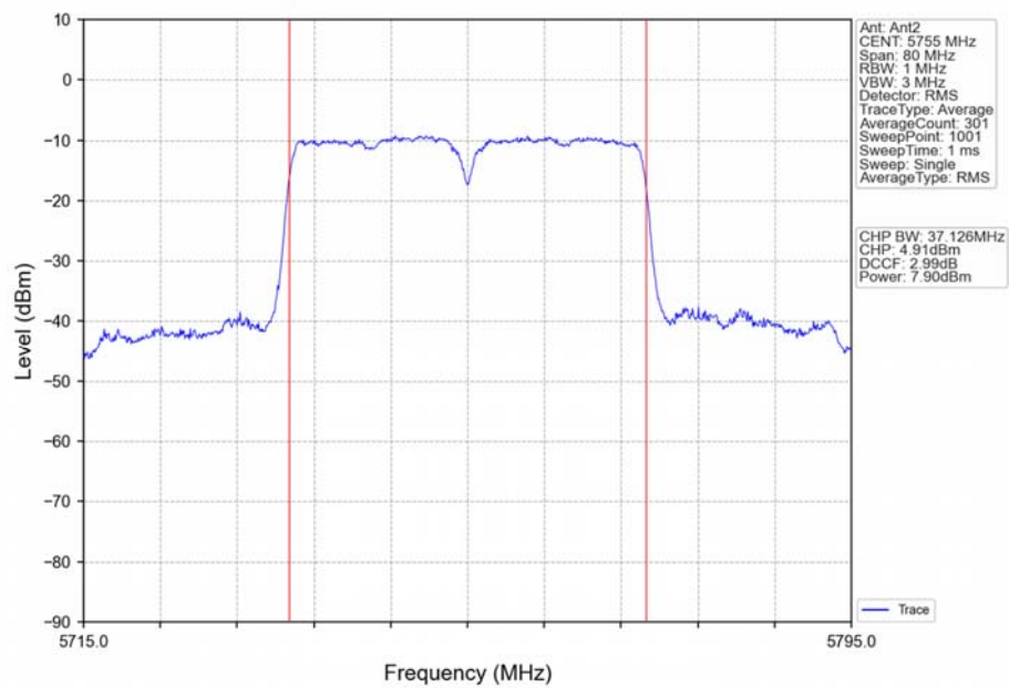
802.11n(HT40)_LCH_5755MHz_Ant2_NTNV
