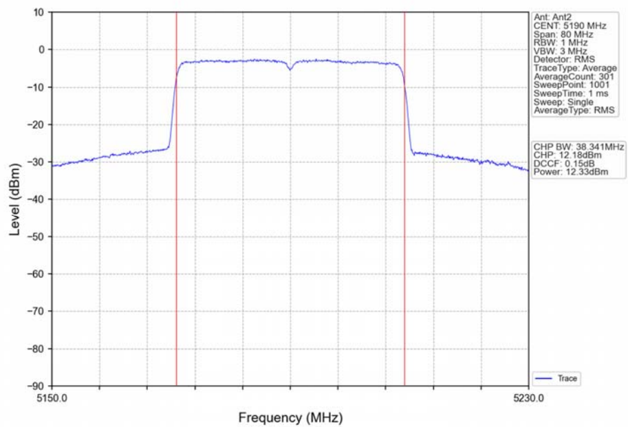
802.11ax(HEW40)_LCH_5190MHz_RU484_Left_Ant2_NTNV
