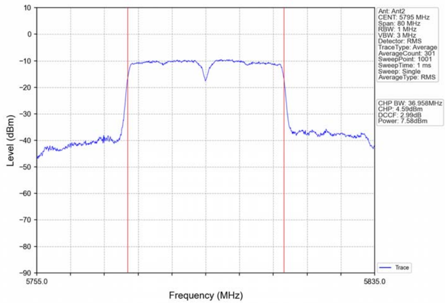
802.11n(HT40)_HCH_5795MHz_Ant2_NTNV
