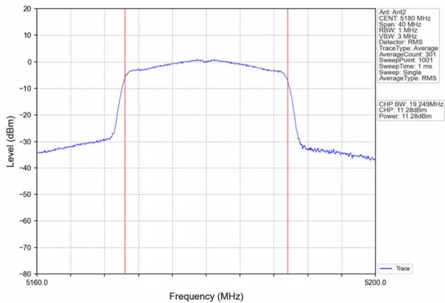
802.11ax(HEW20)_LCH_5180MHz_RU242_Left_Ant2_NTNV
