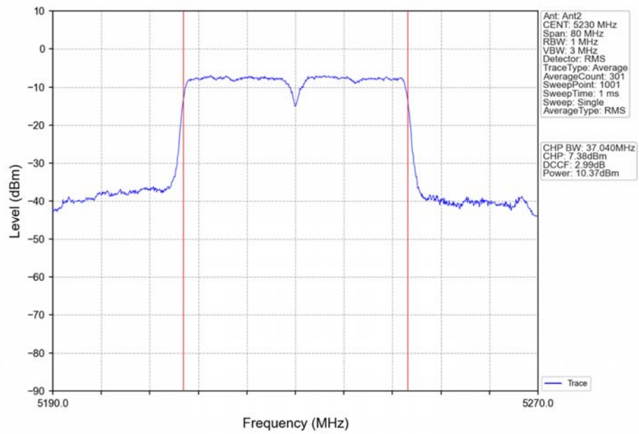
802.11n(HT40)_HCH_5230MHz_Ant2_NTNV
