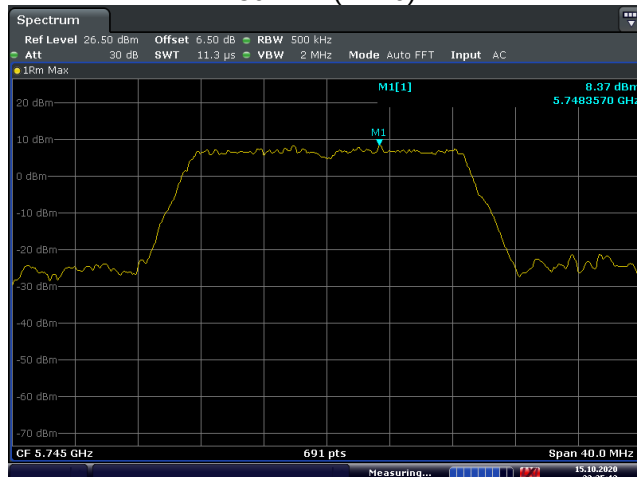
802.11n(HT20)
