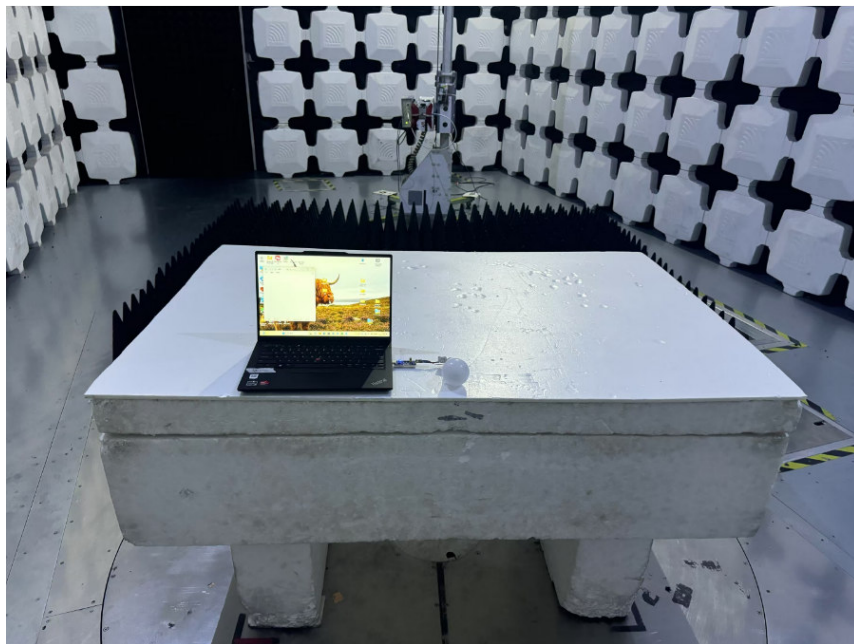
1GHz-18GHz
