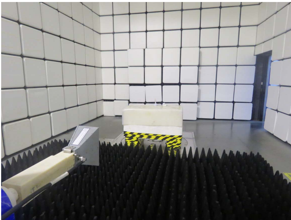
1GHz-18GHz
