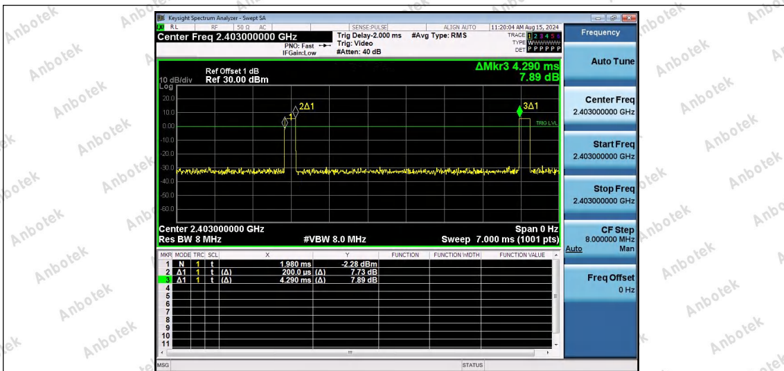
NTNV-2.4G-Ant1-2403
