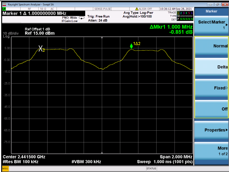
GFSK
