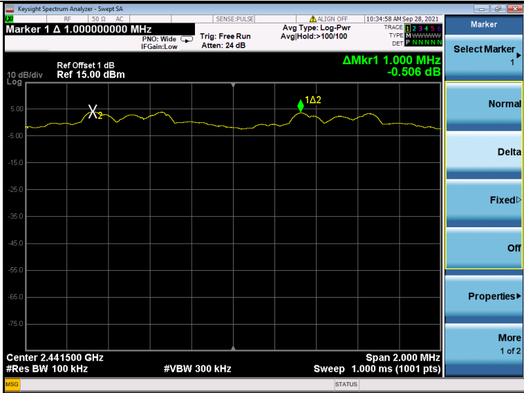
\pi/4 DQPSK
