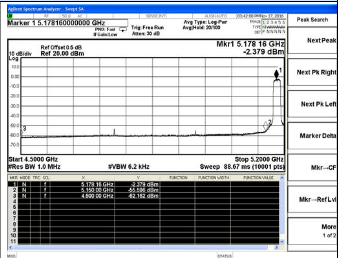
802.11ac20-Low channel(Average)
