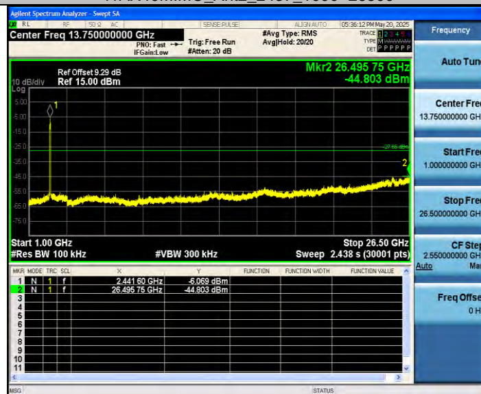
11AX40MIMO_Ant1_2452_0~Reference
