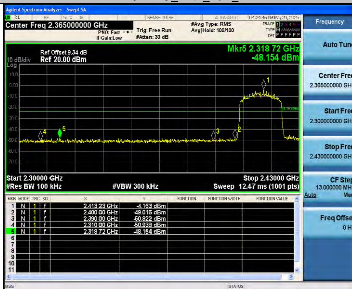
11AX20MIMO_Ant2_Low_2412
