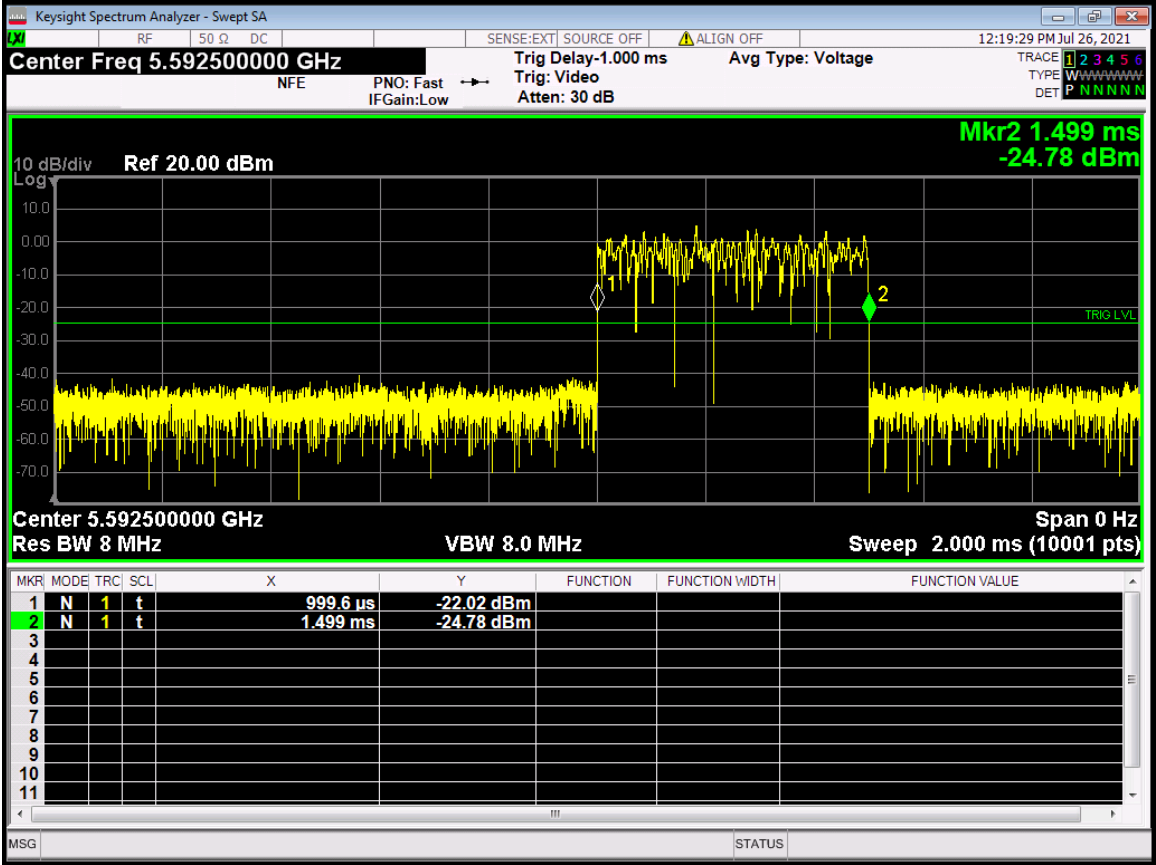
Channel 11 : 5592.5 MHz : On pulses
