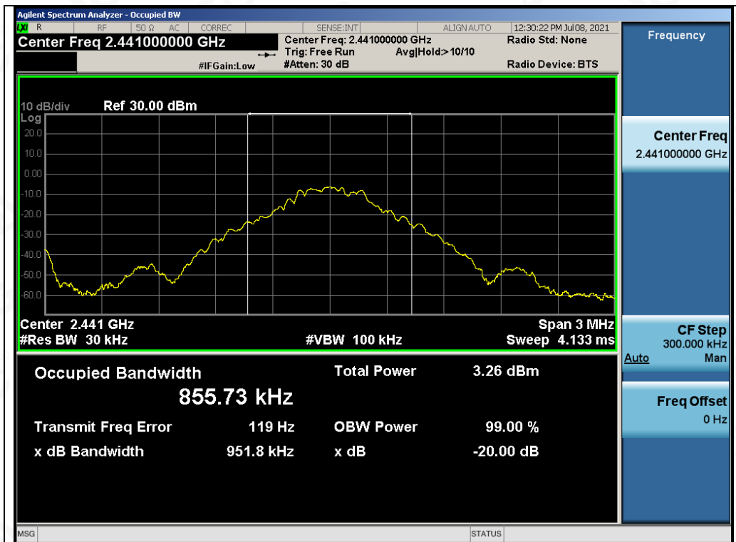
Test_Graph_BR_ANT1_2441_1Mbps_OBW
