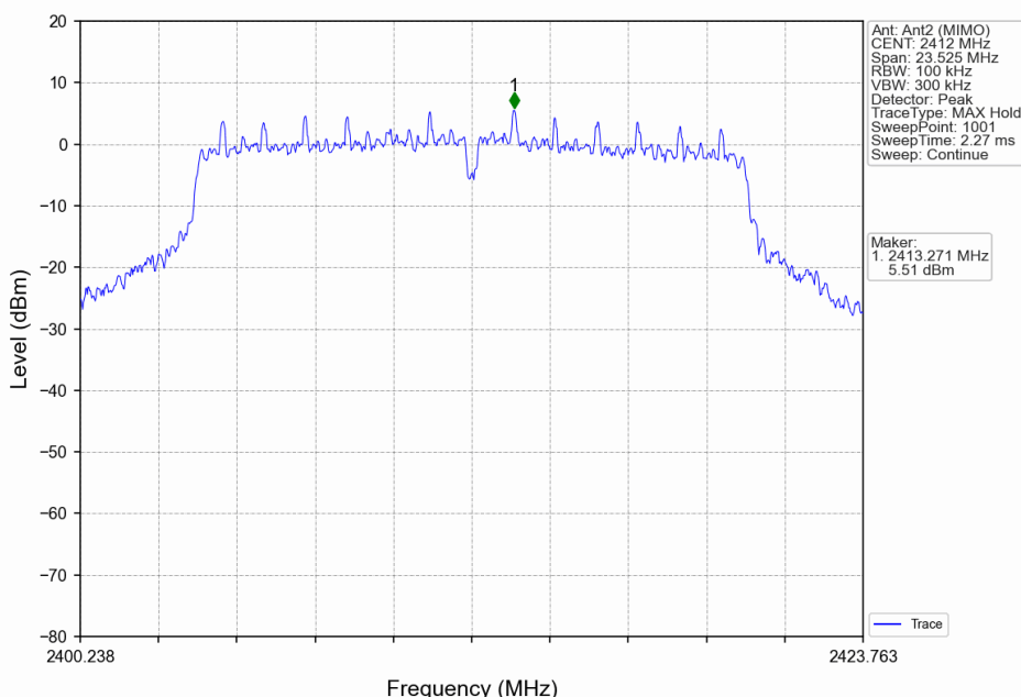
802.11g_LCH_2412MHz_Ant2 (MIMO)_NTNV
