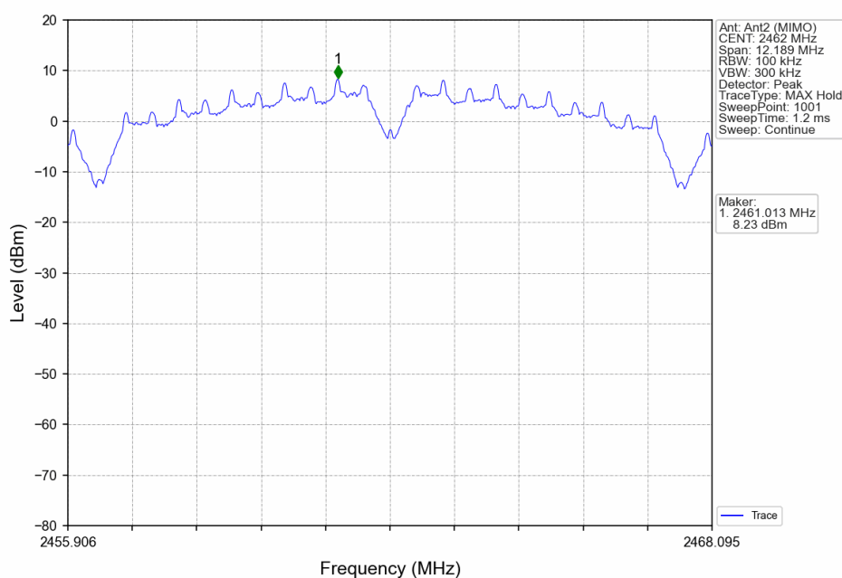
802.11b_HCH_2462MHz_Ant2 (MIMO)_NTNV
