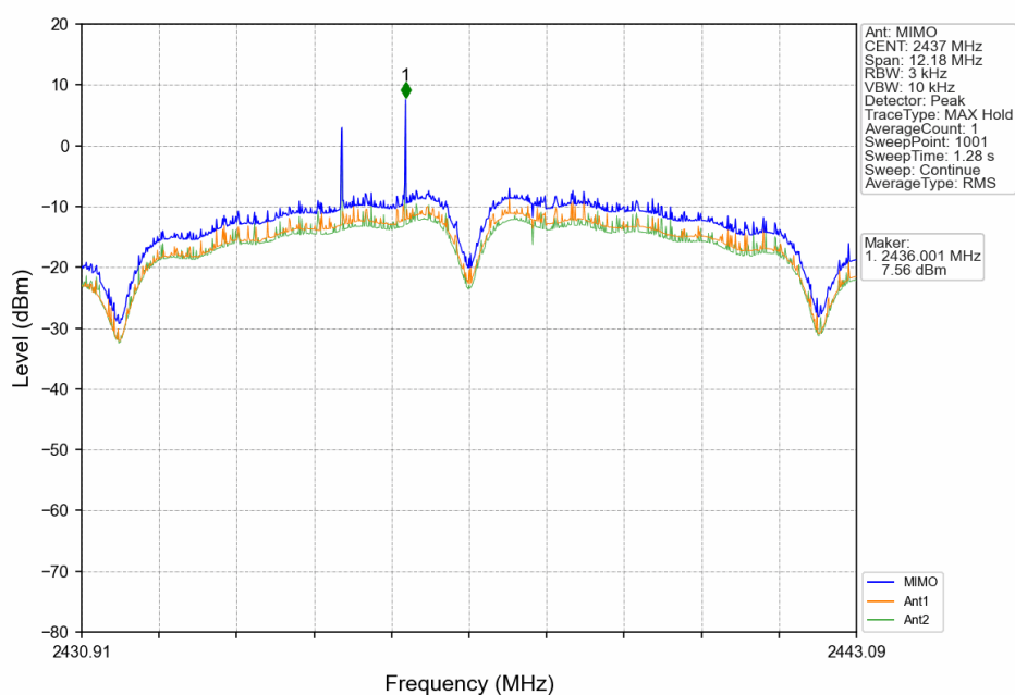
802.11b_MCH_2437MHz_MIMO_NTNV
