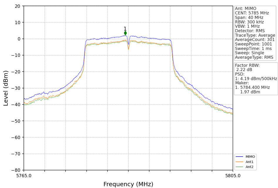
802.11a_MCH_5785MHz_MIMO_NTNV
