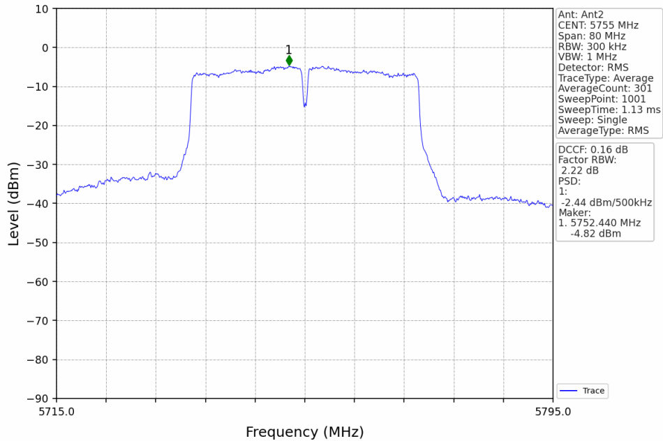
802.11ac(VHT40)_LCH_5755MHz_MIMO_NTNV
